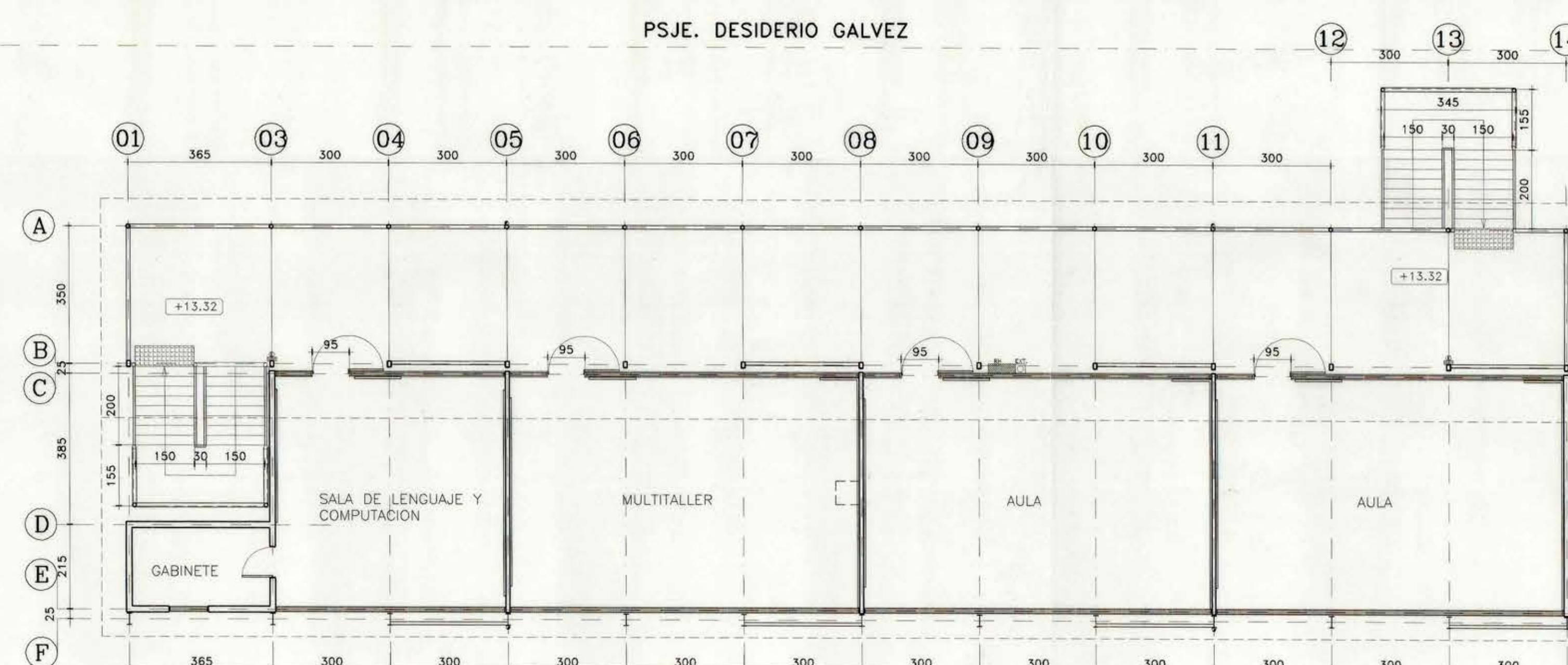
PLANTA 2º NIVEL ESC: 1:100
