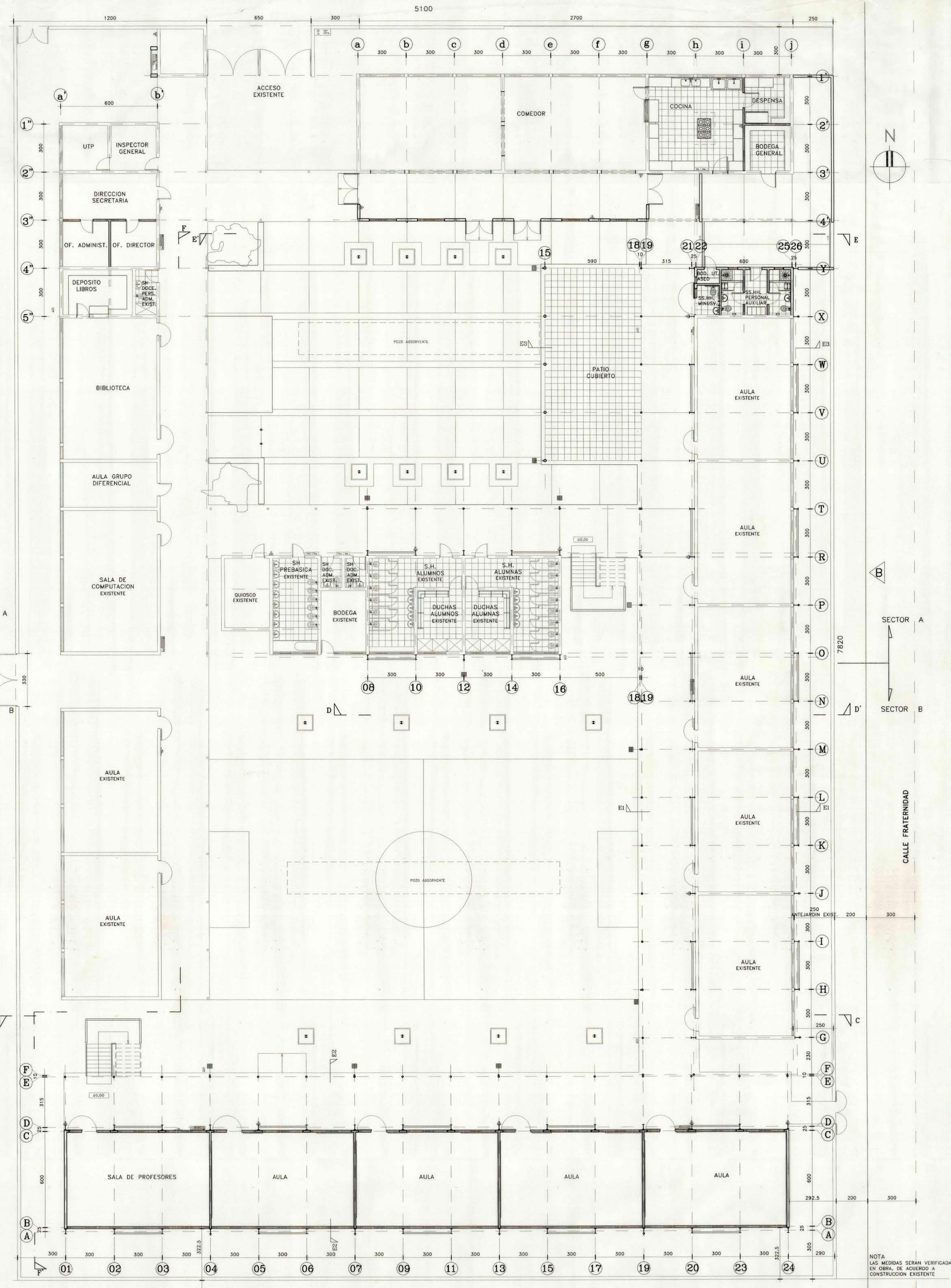
PLANTA GENERAL 1º NIVEL ESCALA: 1:100
