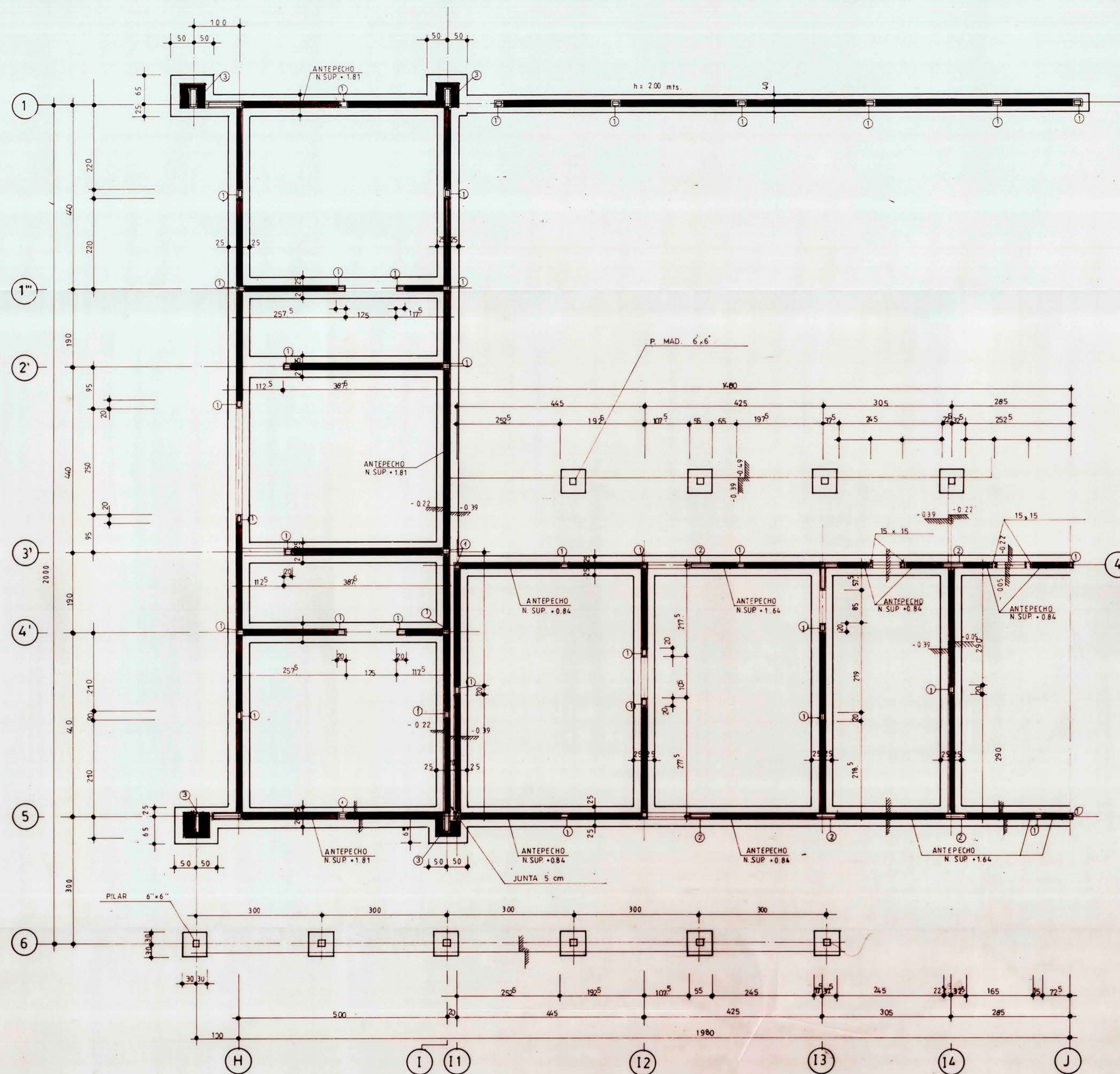
PLANTA DE FUNDACIONES
