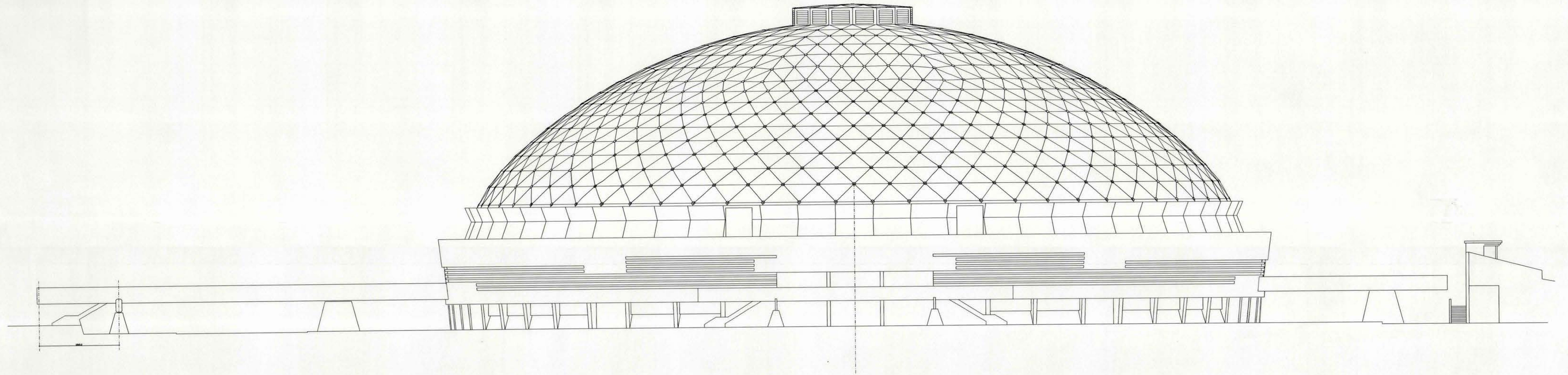
ELEVACION SUR CUPULA ESCALA 1:250
