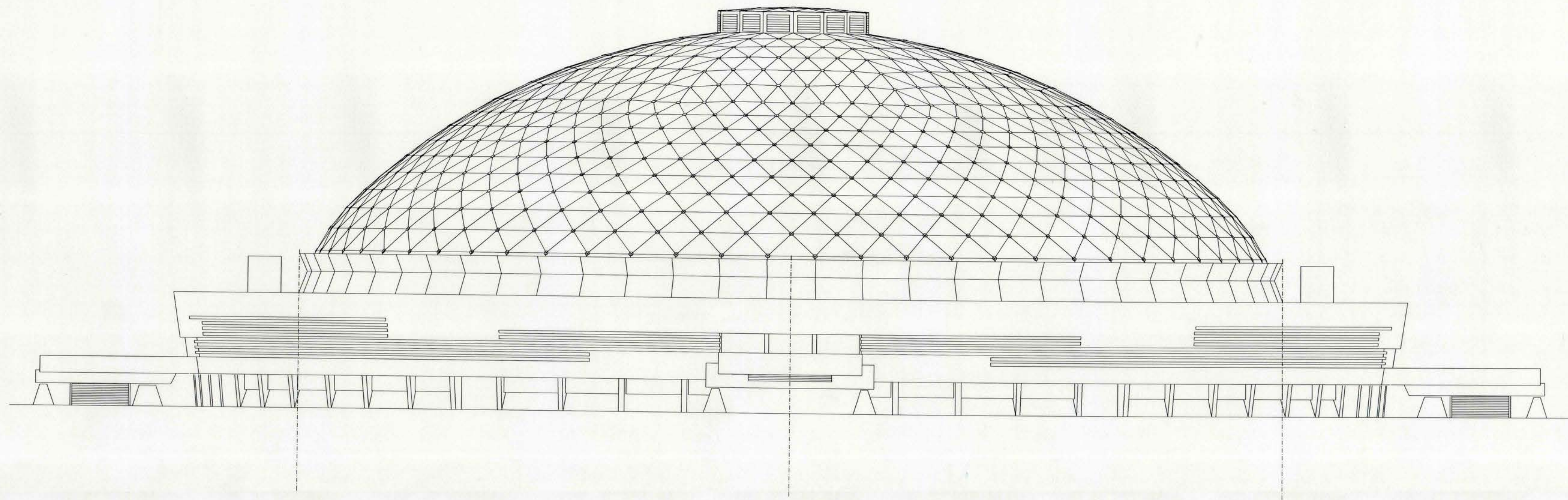
ELEVACION ORIENTE
