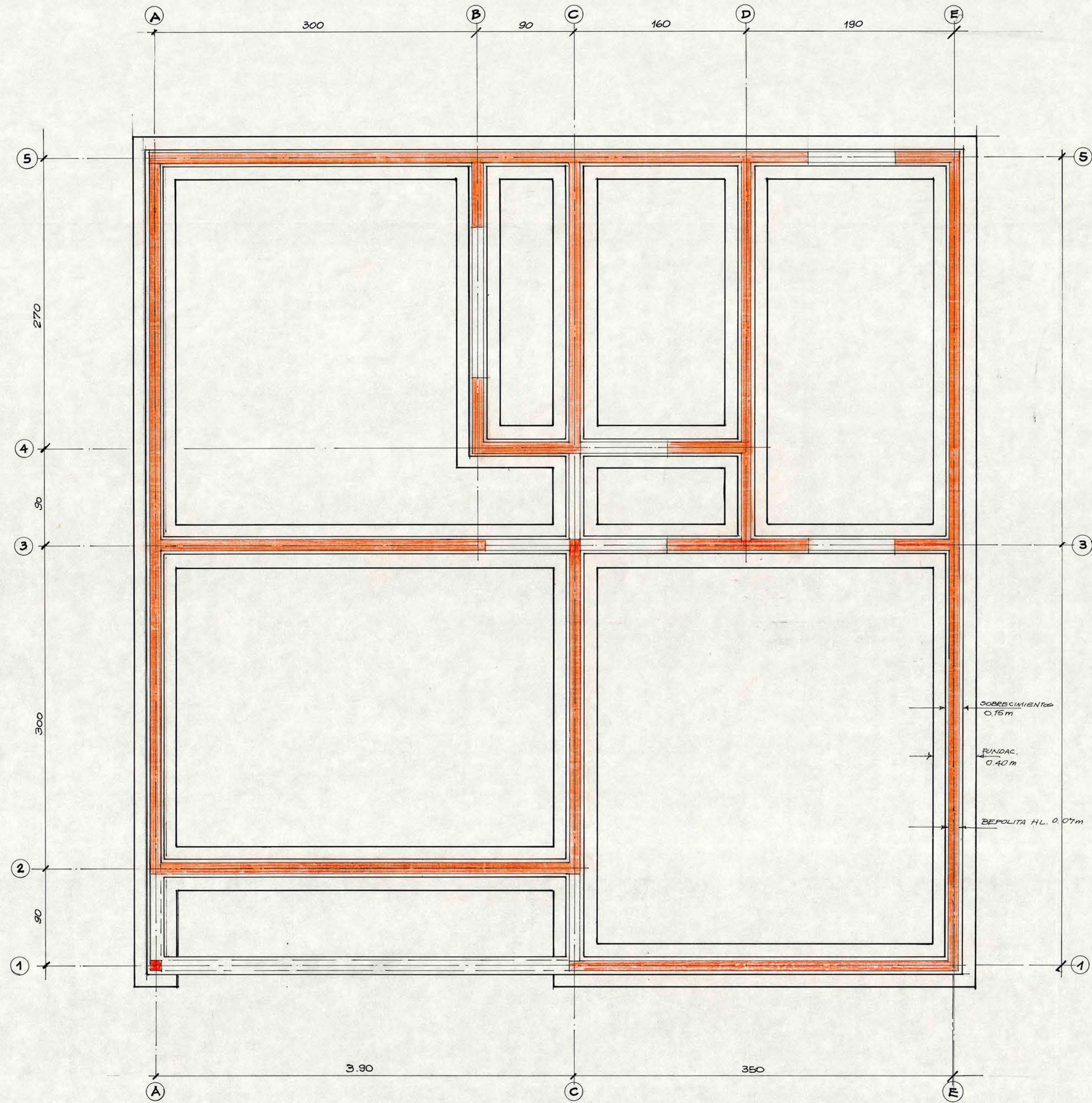
PLANTA FUNDACIONES
