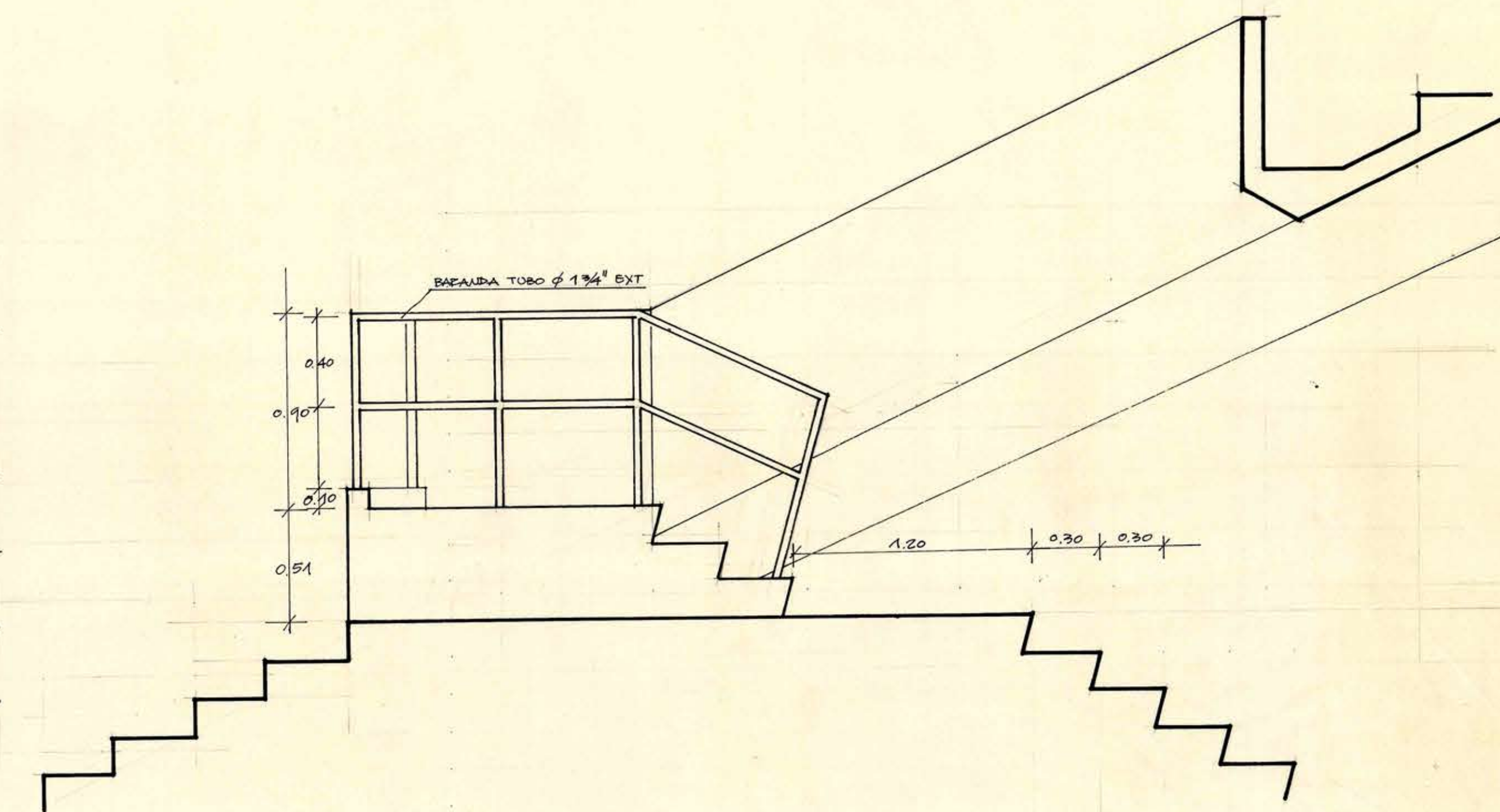
CORTE S/B-B'
