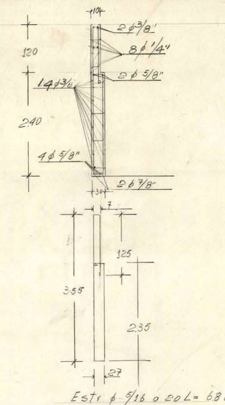
Corte Marco de Fachada (por la clave)
