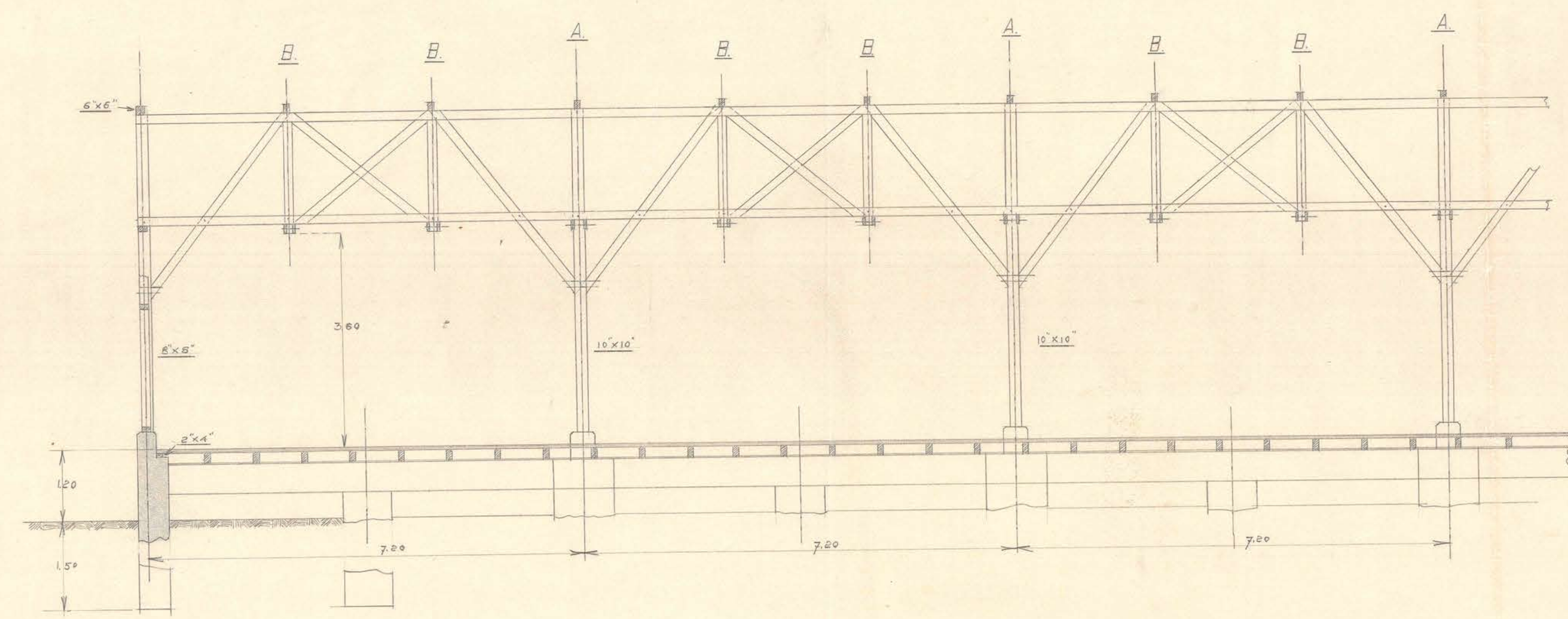
CORTE LONGITUDINAL
