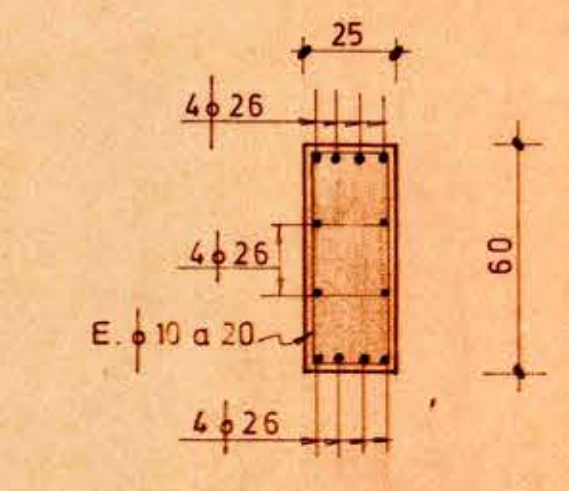
PILAR P2 Esc. 1:20
