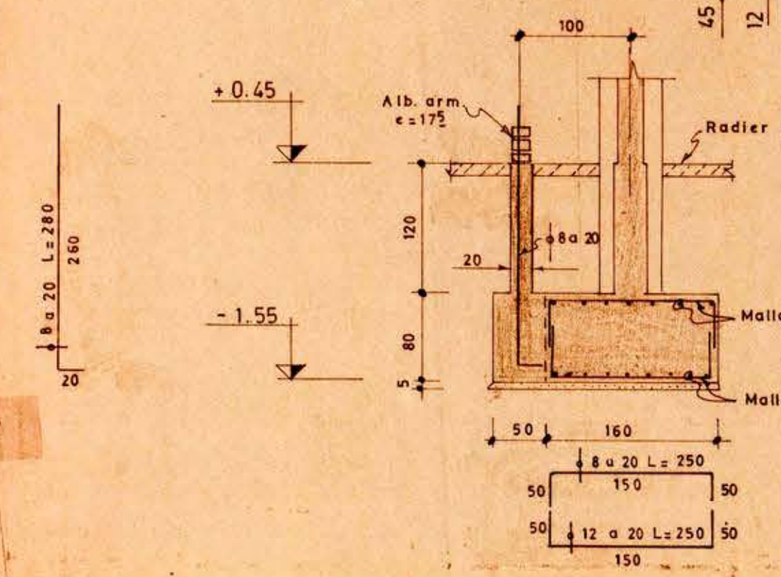
Corte E Esc. 1:30
