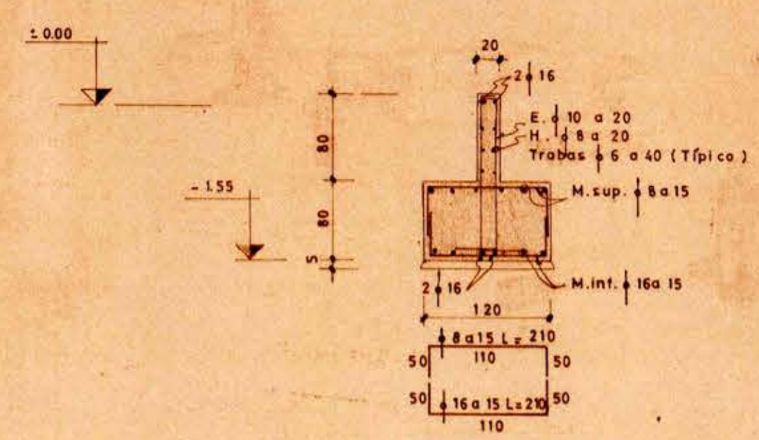
Corte D Esc. 1:30
