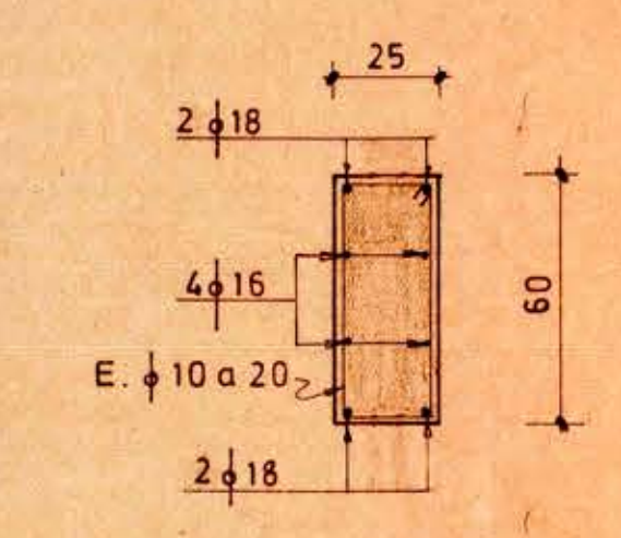
PILAR P5 Esc. 1:20
