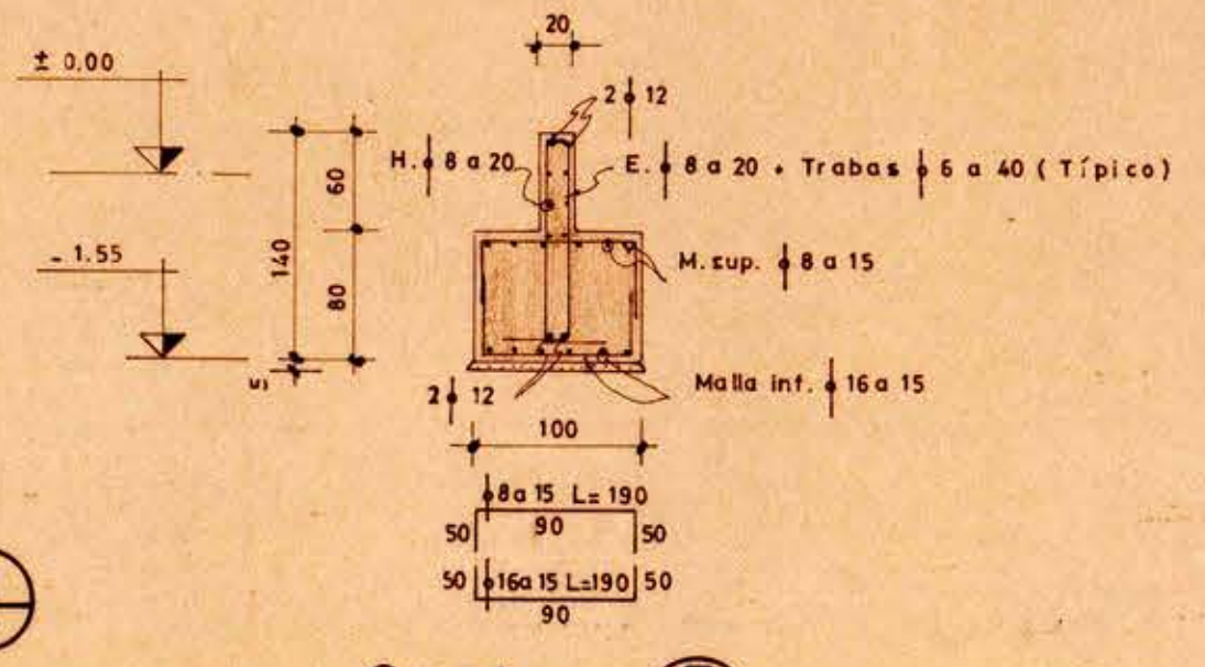
Corte F Esc. 1:30
