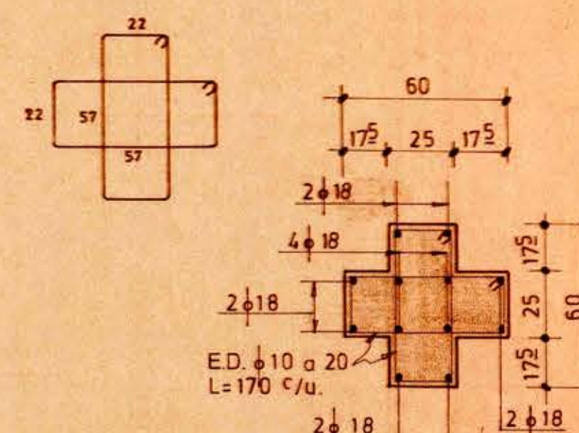
PILAR P3 Esc. 1:20
