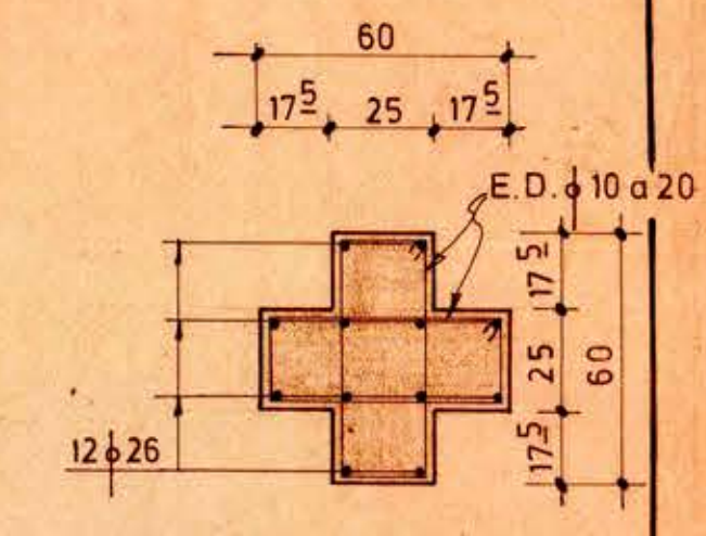
PILAR P1 Esc. 1:20
