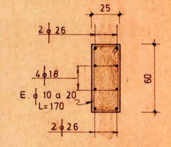
PILAR P4 Esc. 1:20
