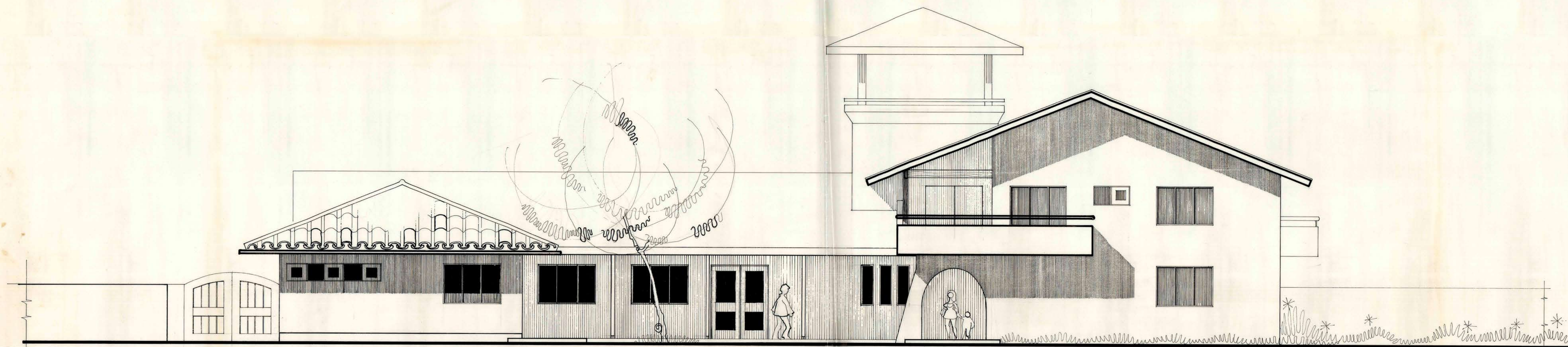
FACHADA PRINCIPAL (PONIENTE) escala 1/50.
