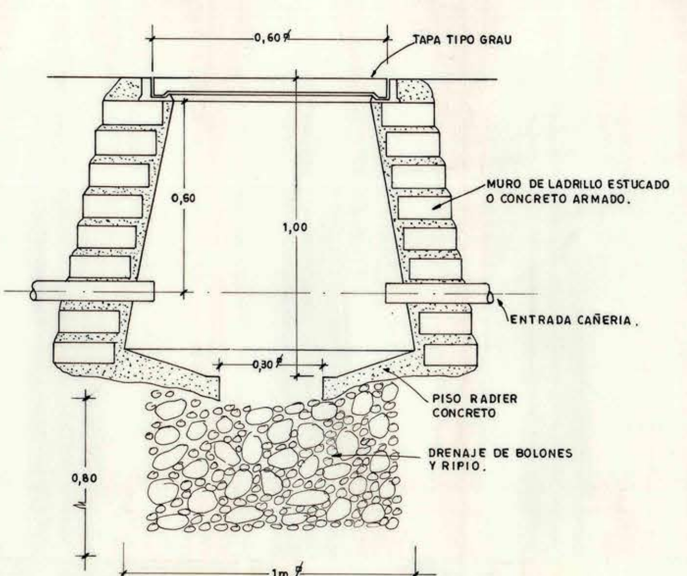
CAMARA TIPO PARA CANALIZACION SUBTERRANEA. SIN ESCALA
