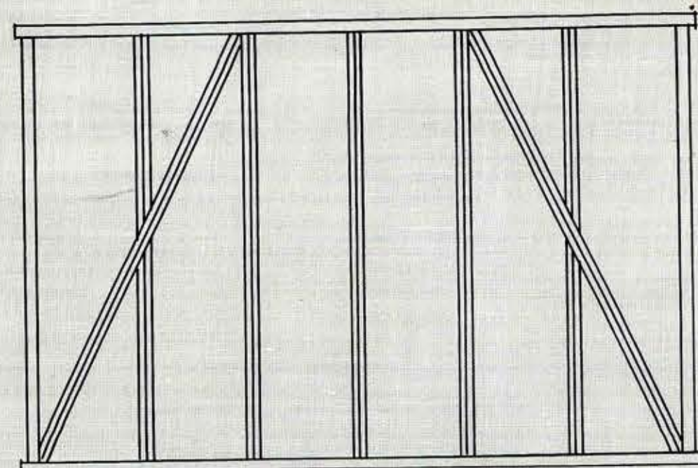
Tabique lateral.
