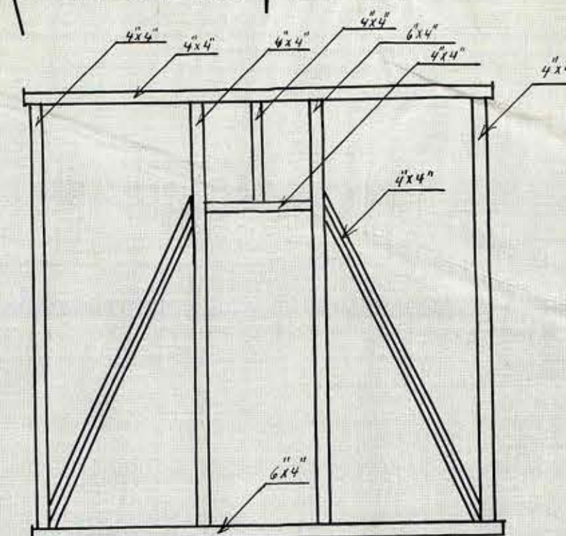
Tabique oficina.
