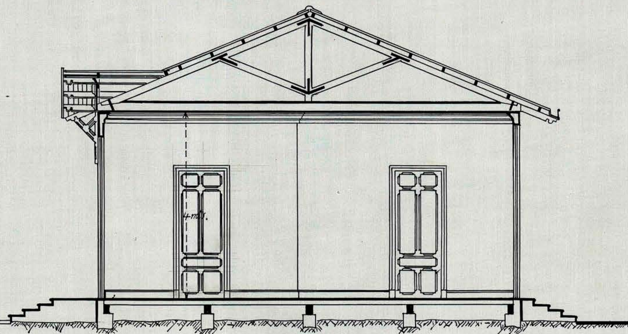
— CORTE —
