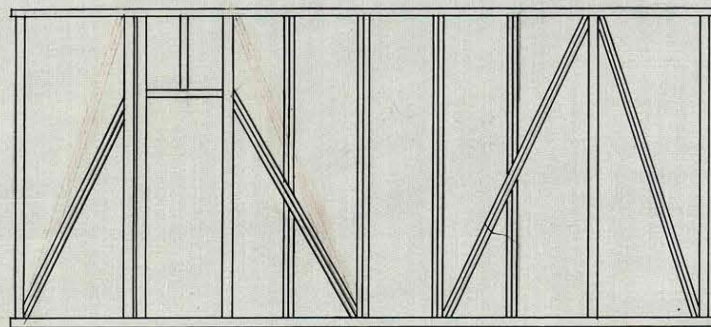
Tabique sala de clase (interior)
