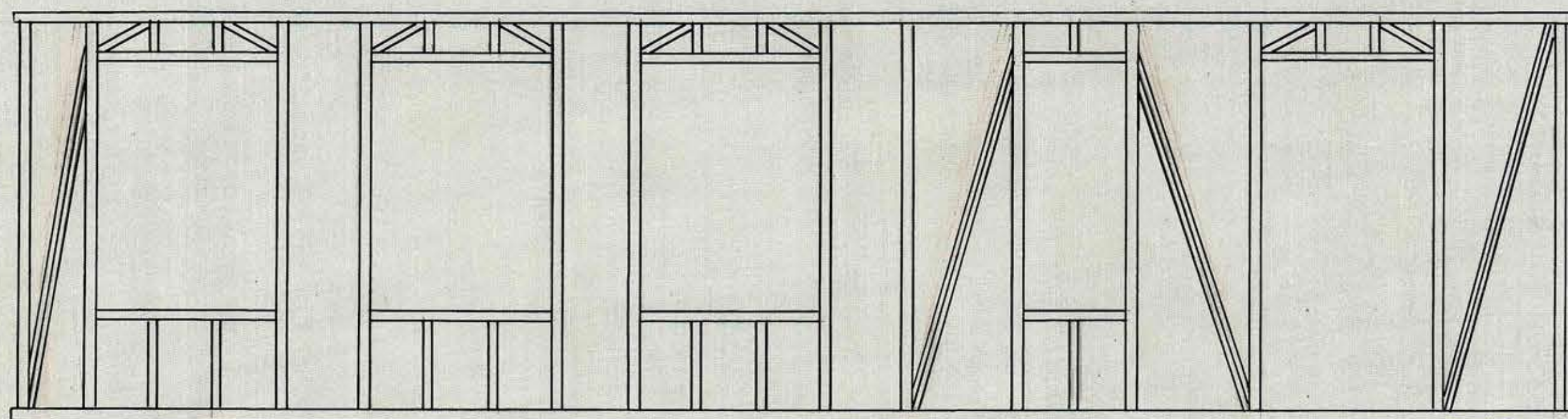
Tabique fachada principal.
