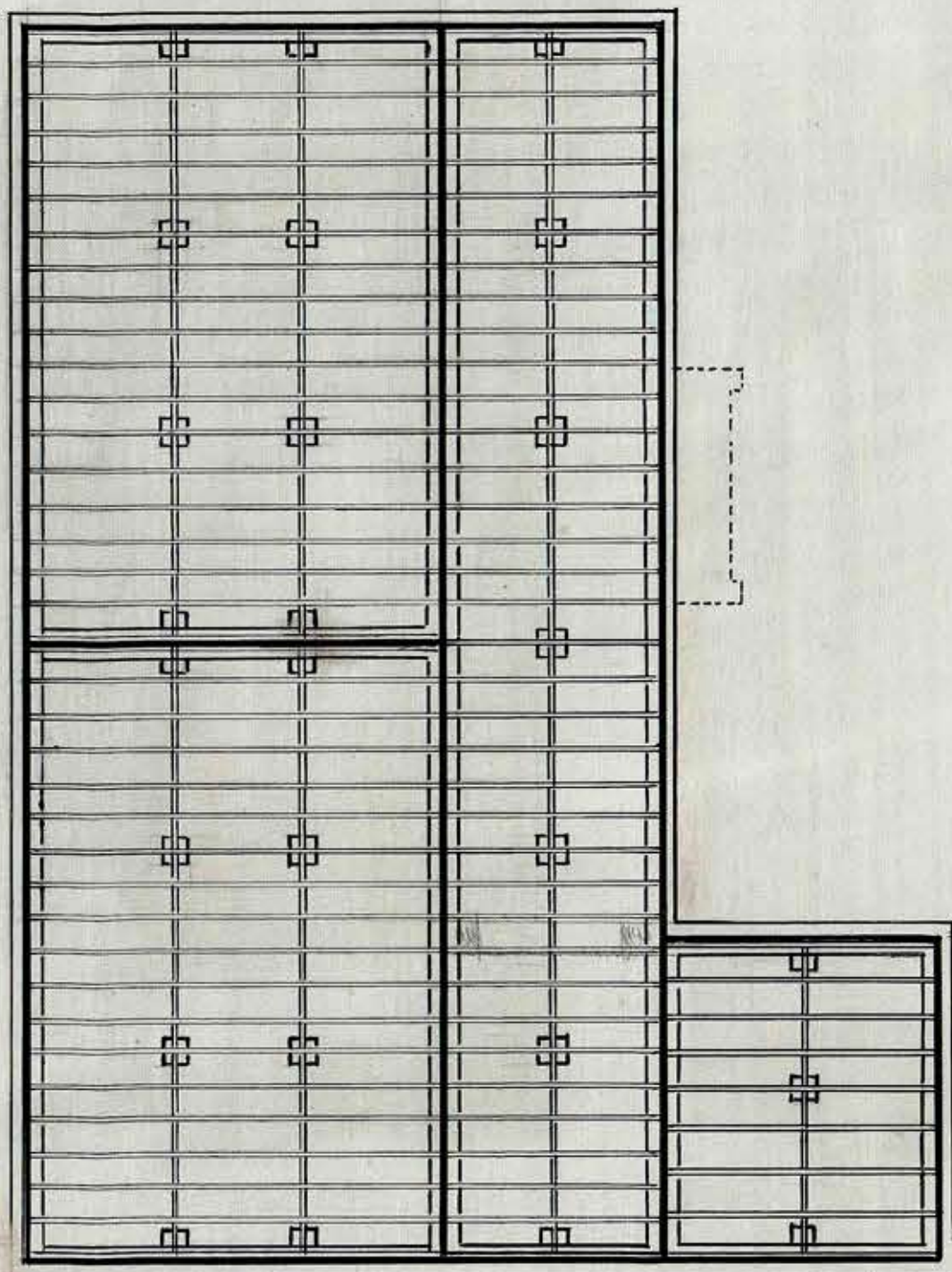
Cimientos y Envigados
