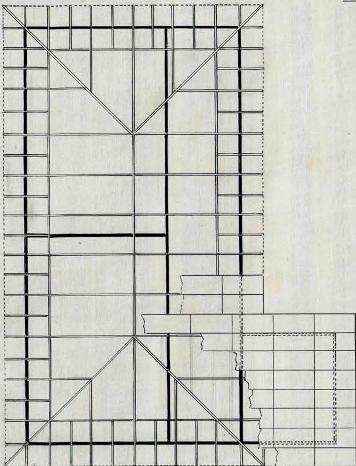
Enmaderaciones de la Techumbre
