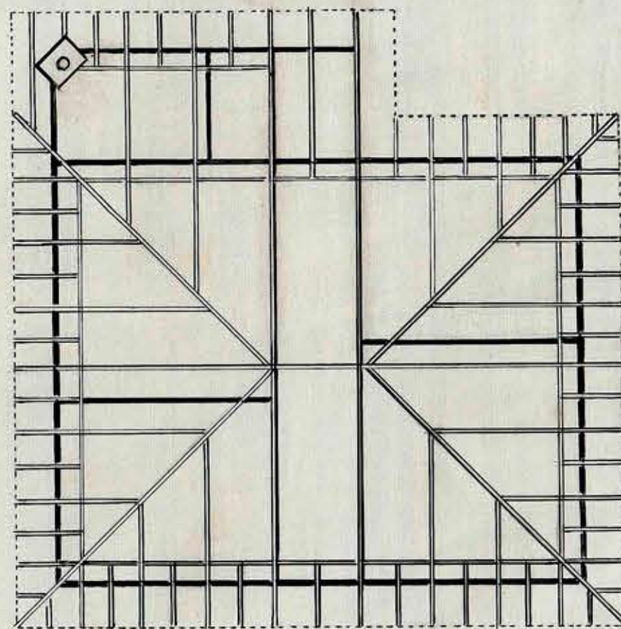
Enmaderaciones de la Techumbre
