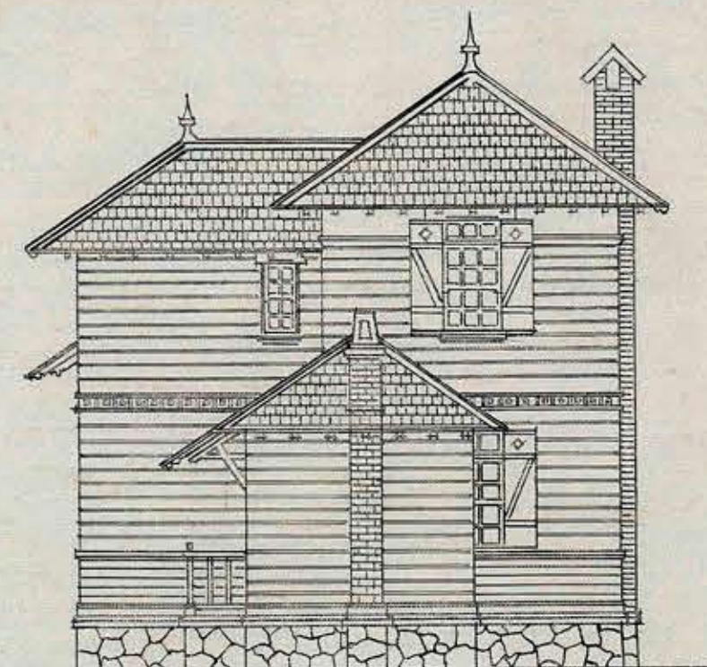
FACHADA POSTERIOR
