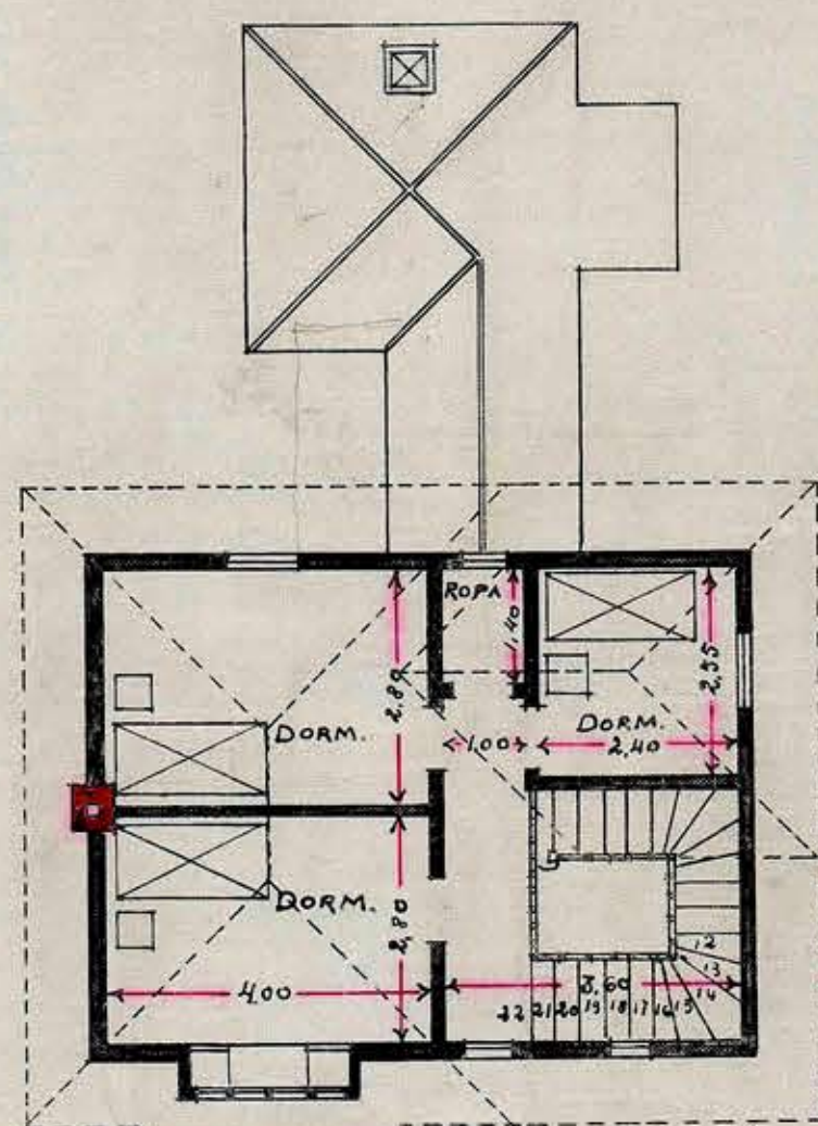
SEGUNDO PISO
