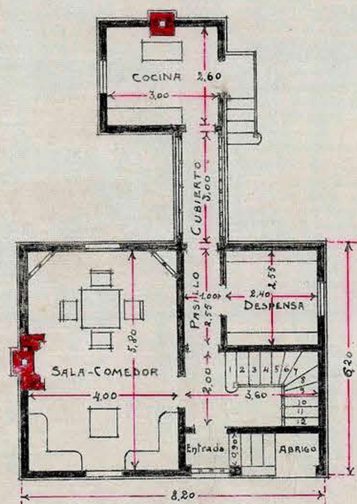
PRIMER PISO
