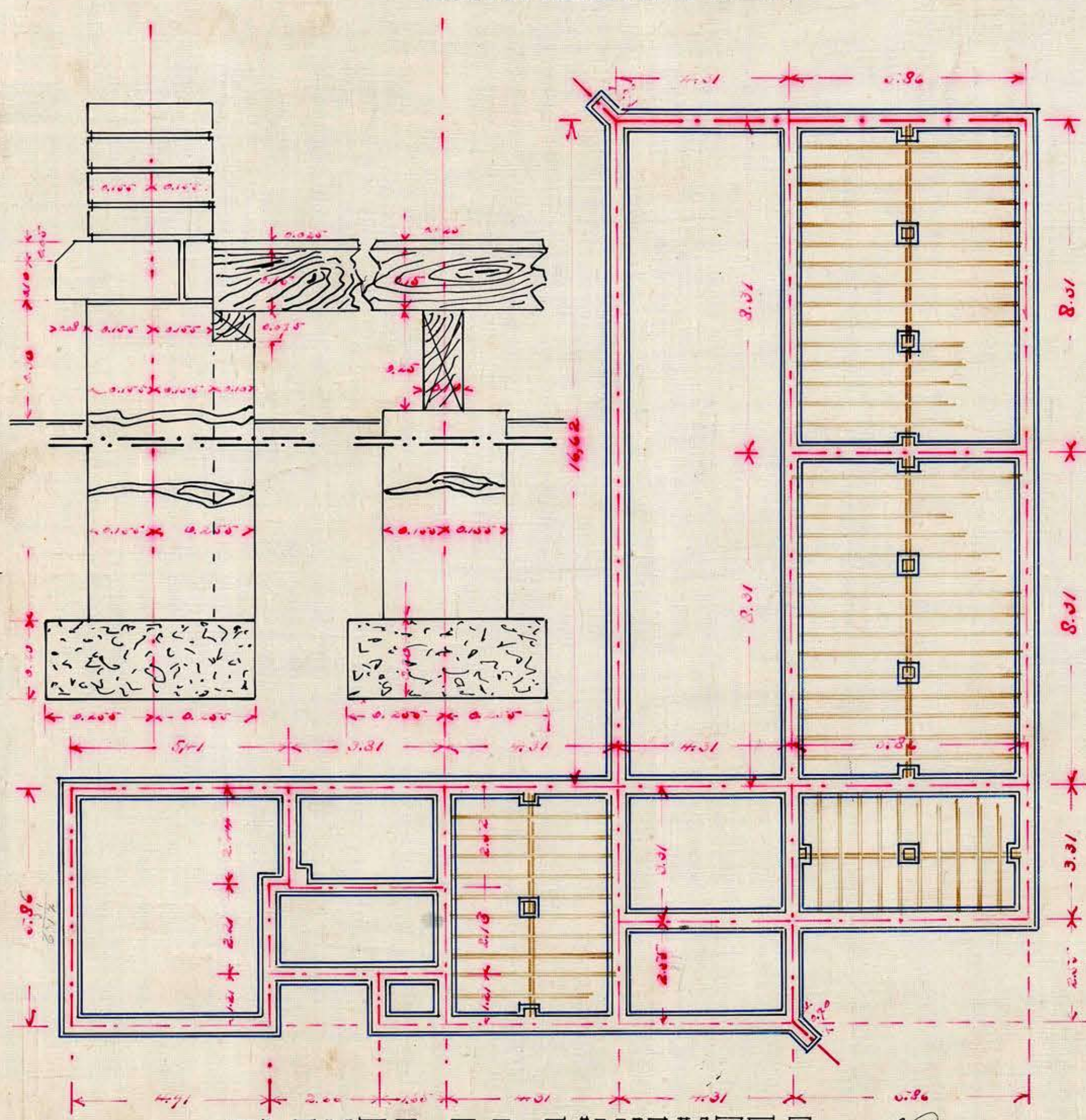
PLANTA DE CIMIENTOS
