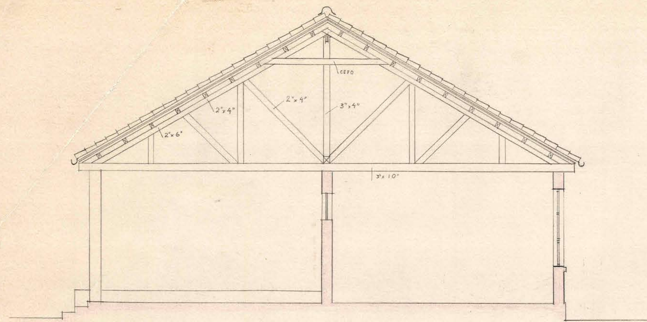
CORTE AA'
