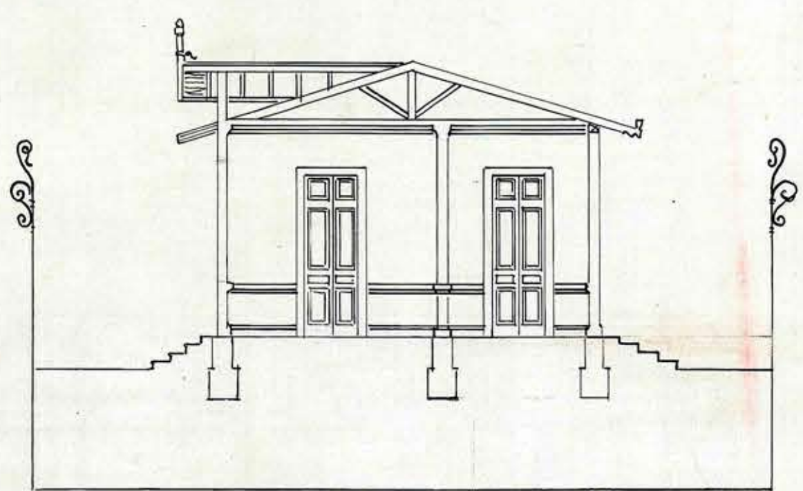
SECCION LONGITUDINAL
