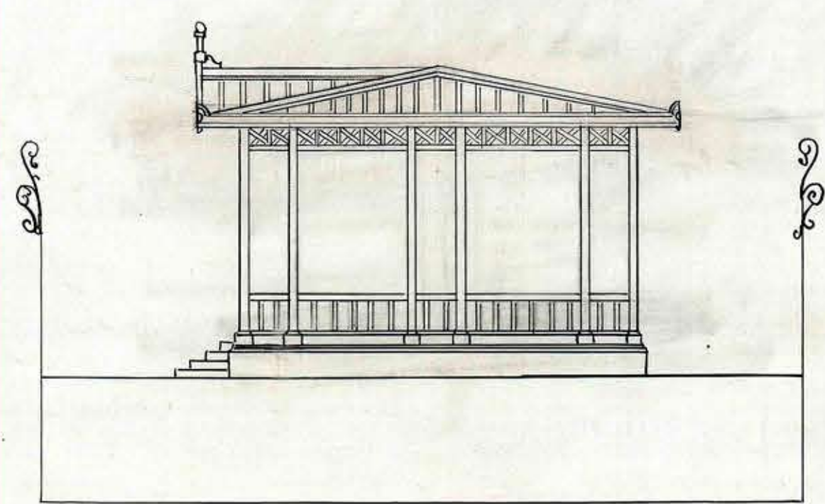
FACHADA LATERAL
