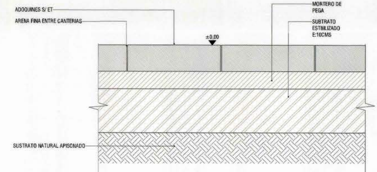
DETALLE DE ADQUINES TIPO 1:5
