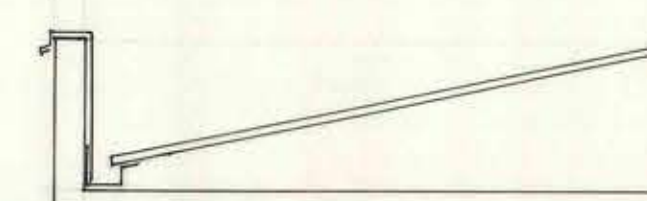
TIPO C.F. = CANAL FORRO CORTAGOTERA EN REMATE DE ANTETECHOS
