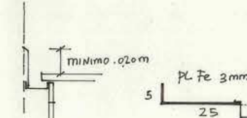
TIPO C.P.L. = CANAL DE PLANCHA DE FE 3mm doblada DESARROLLO 0.35 m. SOLDADA A VIGUETA LONGITUDINAL DE PATIO Y PASILLO CUBIERTO - DEBE INCLUIR PERFORACIONES RECTANGULARES PARA VENTILACION CON BAJADAS - CUANDO ESTA CANAL PASA ARREGLADA AL PARAMENTO DE UN EDIFICIO, CONSULTAR FORRO SEGUN ESQUEMA
