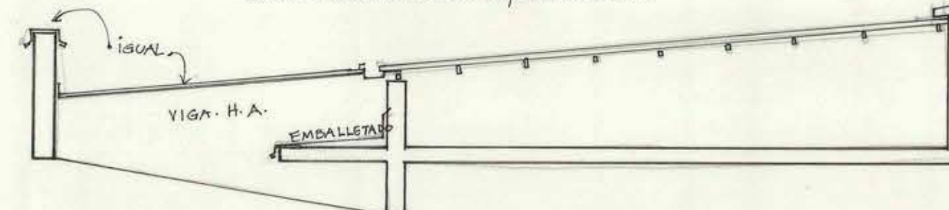
TIPO E.C.F.B2 = COMBINACION DE EMBALLETADO CON CANAL Y FORRO CORTAGOTERAS EN ALERO ADMINISTRACION-BIBLIOTECA
