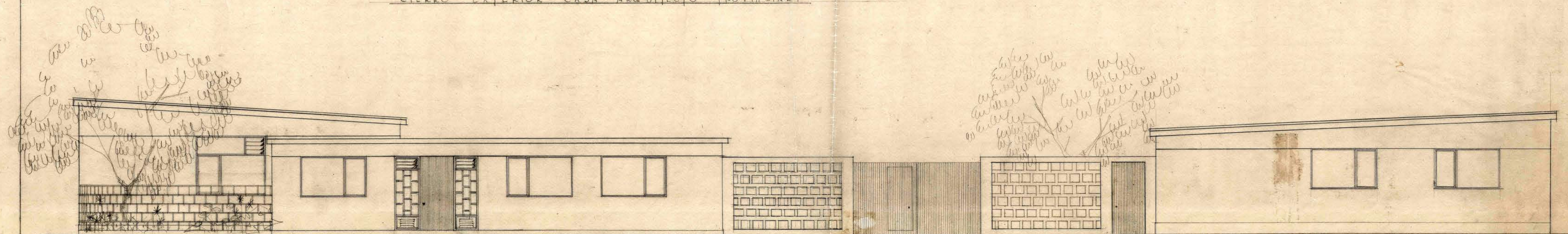
FACHADA POR CALLE 21 DE MAYO
