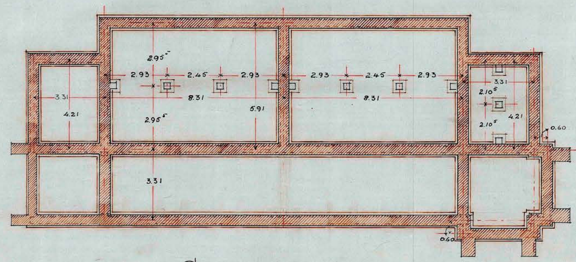
CIMENTOS
