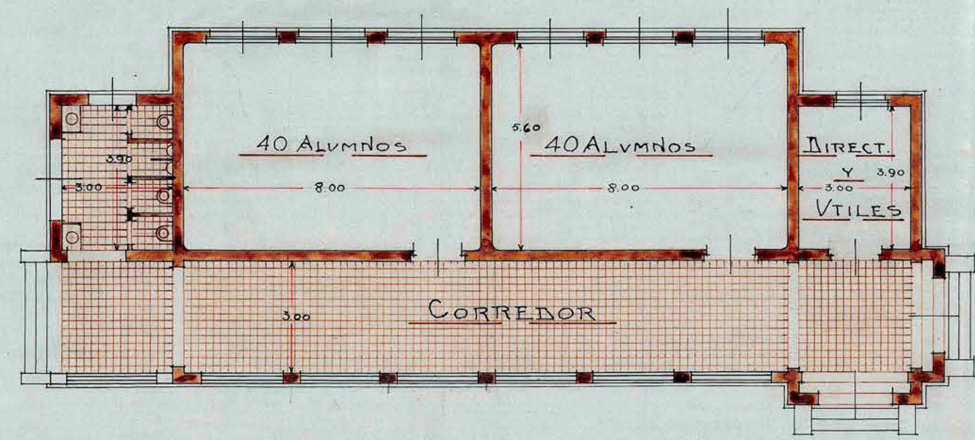
PLANTA
