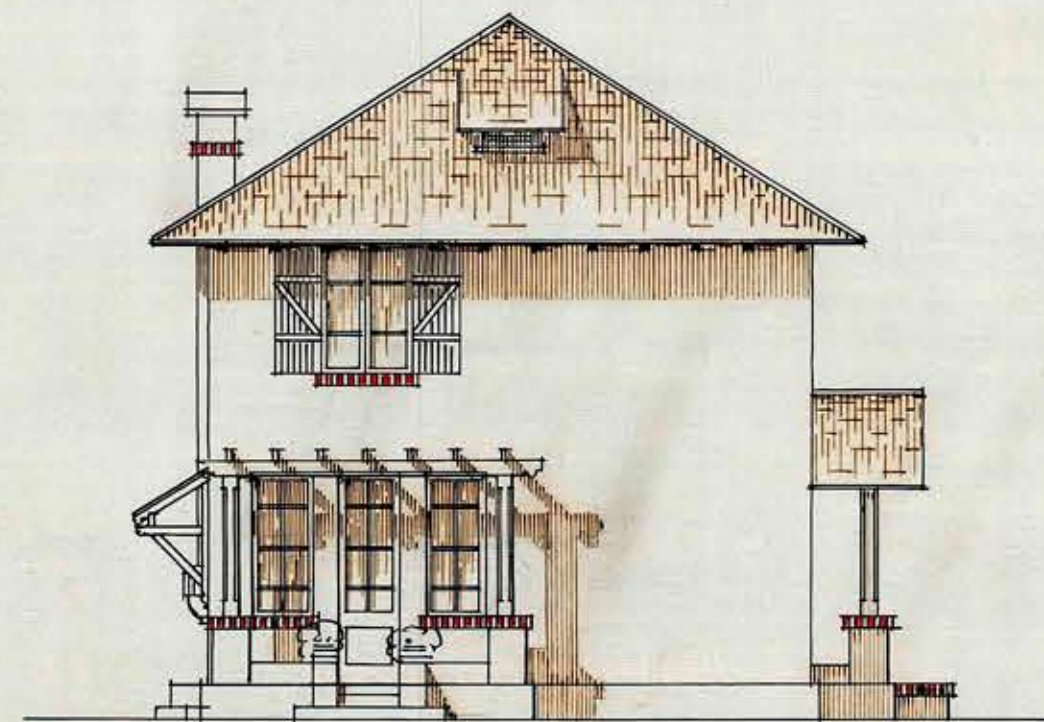
FACHADA ESTE
