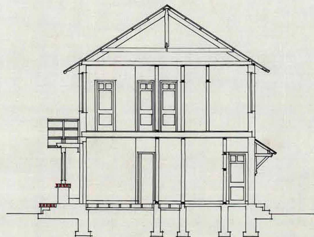
CORTE
