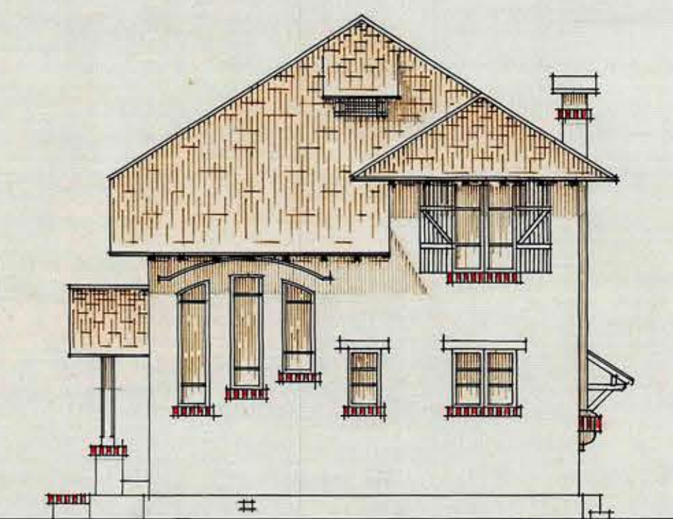
FACHADA OESTE
