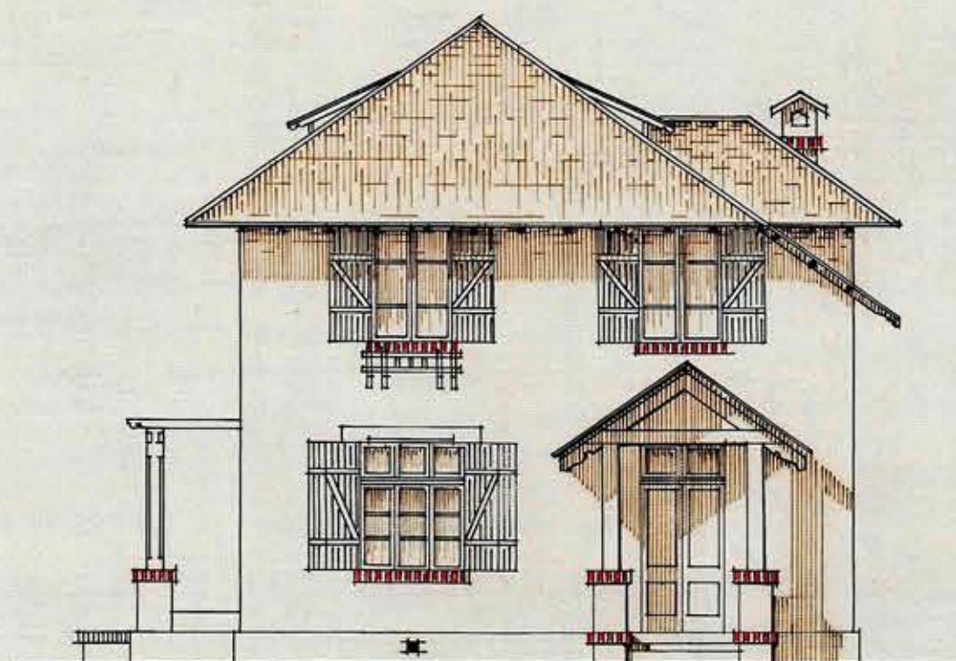
FACHADA NORTE
