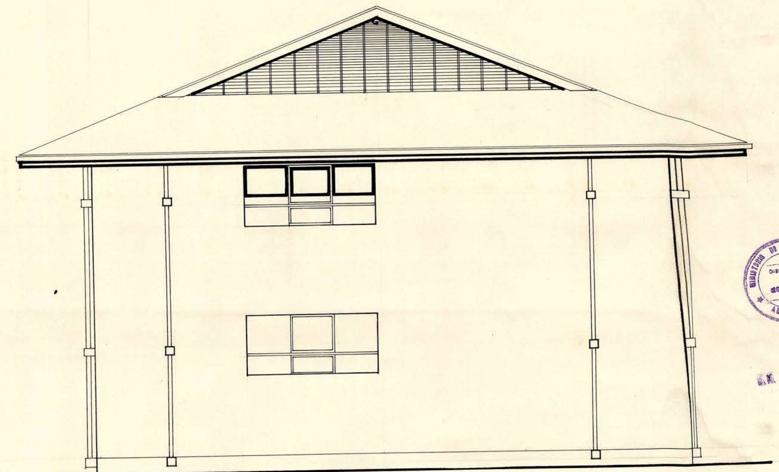
ELEVACION NORTE
