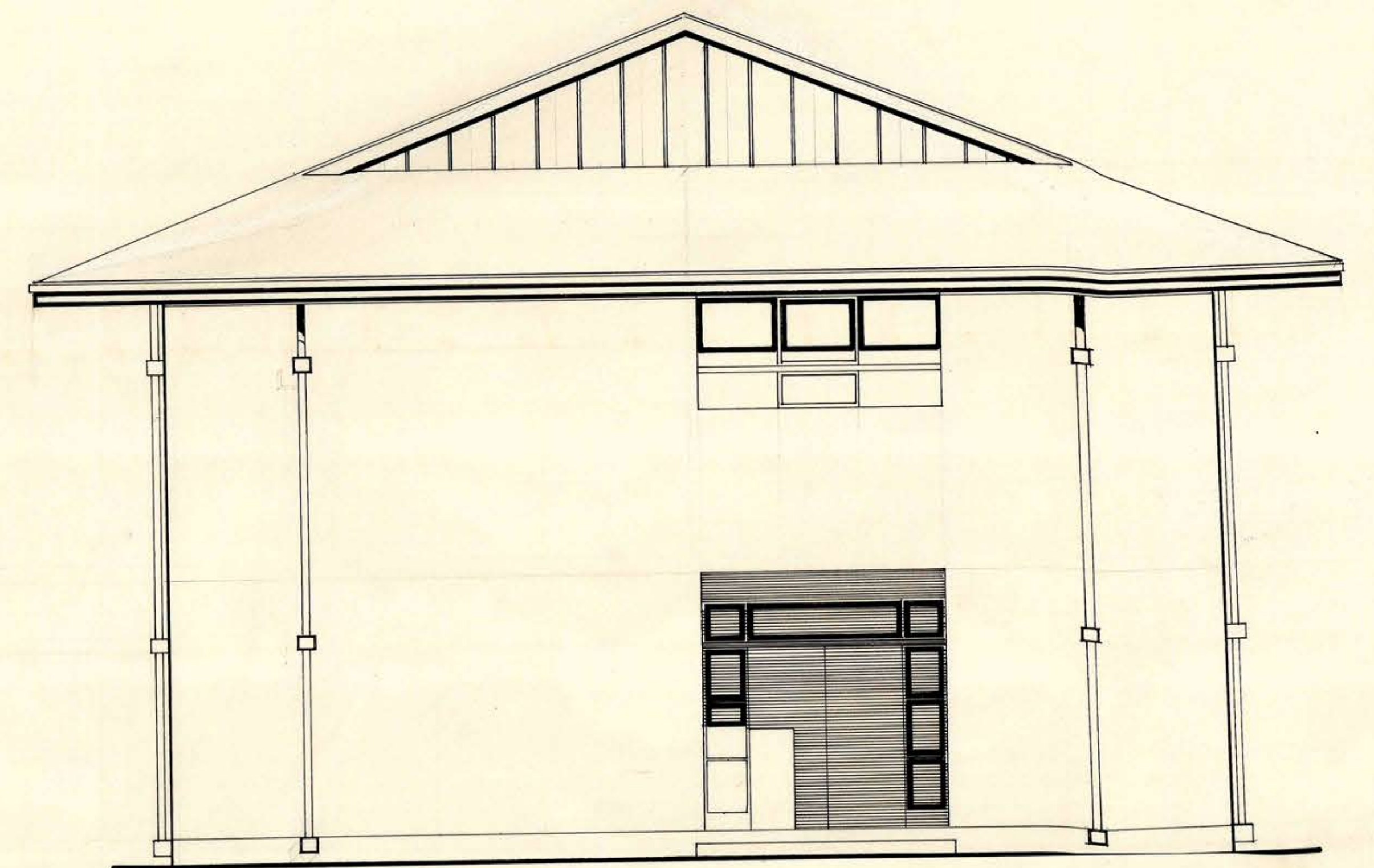
ELEVACION SUR
