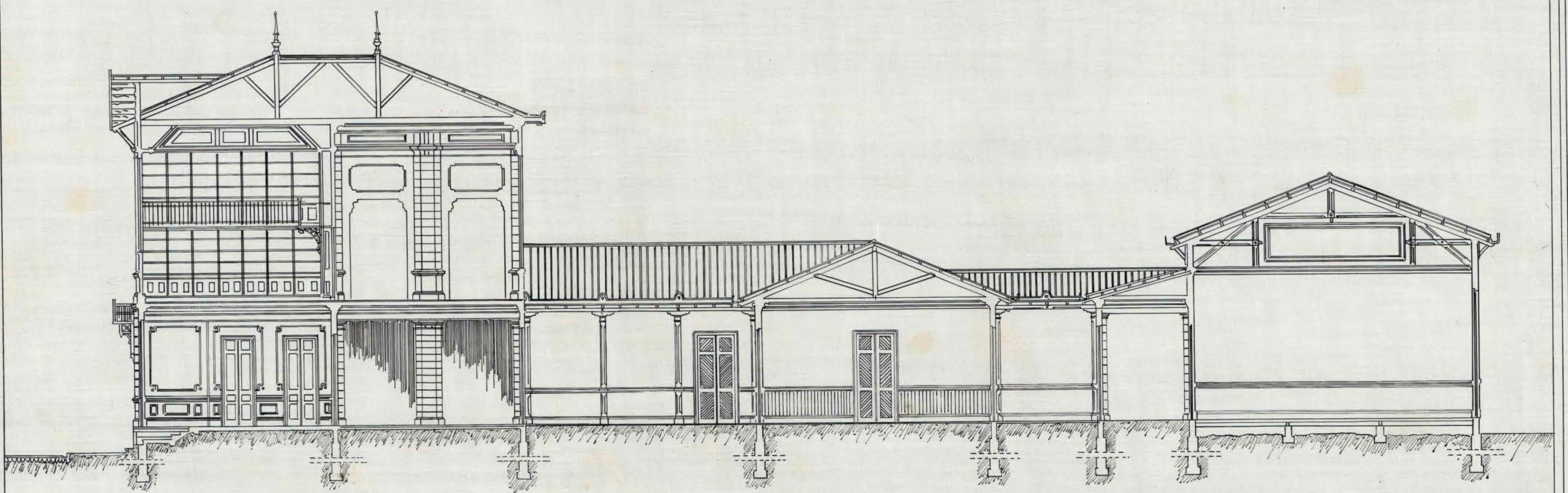
SECCION LONGITUDINAL
