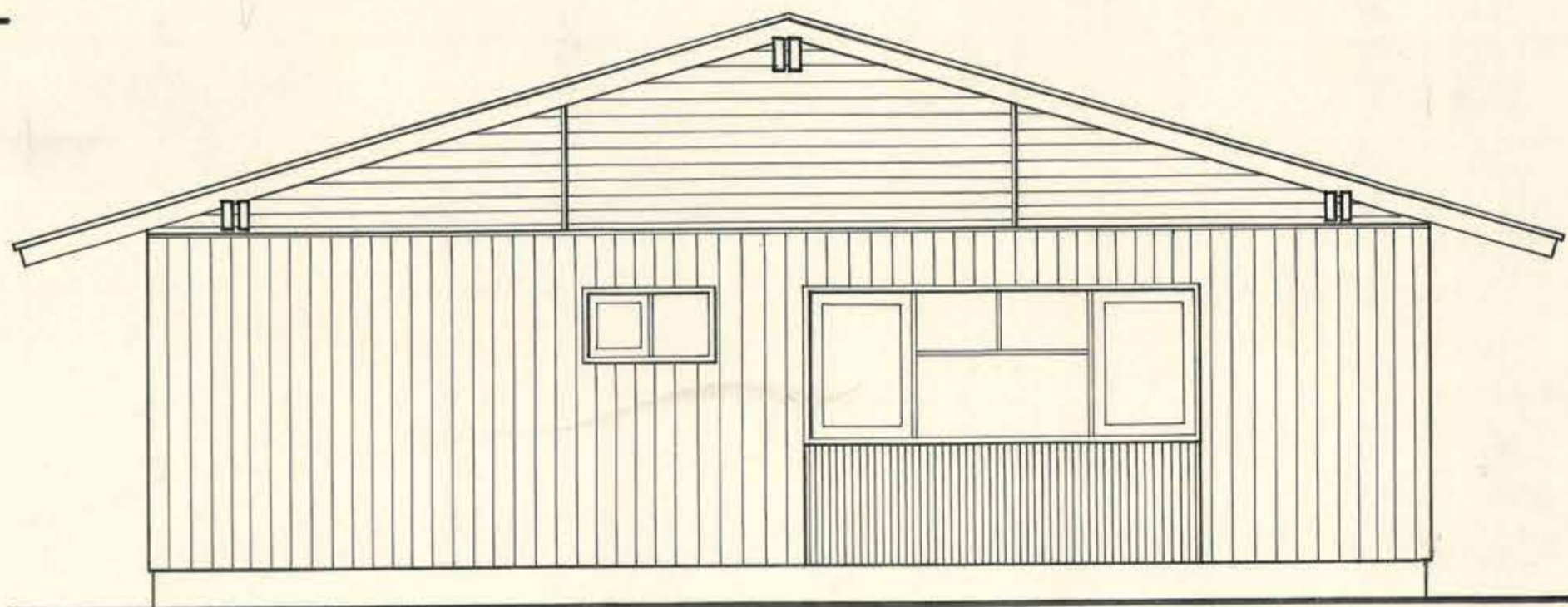
ELEVACION NOR-PONIENTE
