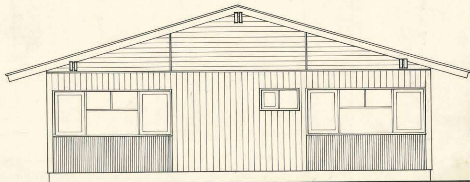
ELEVACION SUR-ORIENTE
