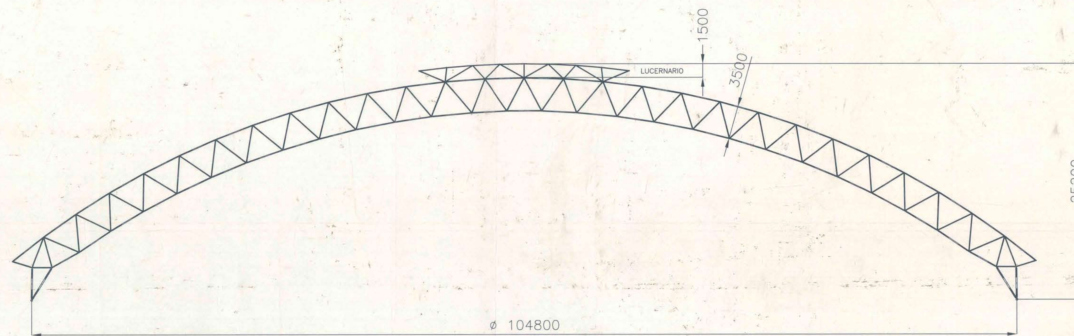
CORTE TIPO GEOMETRIA CUPULA ESCALA 1: 200
