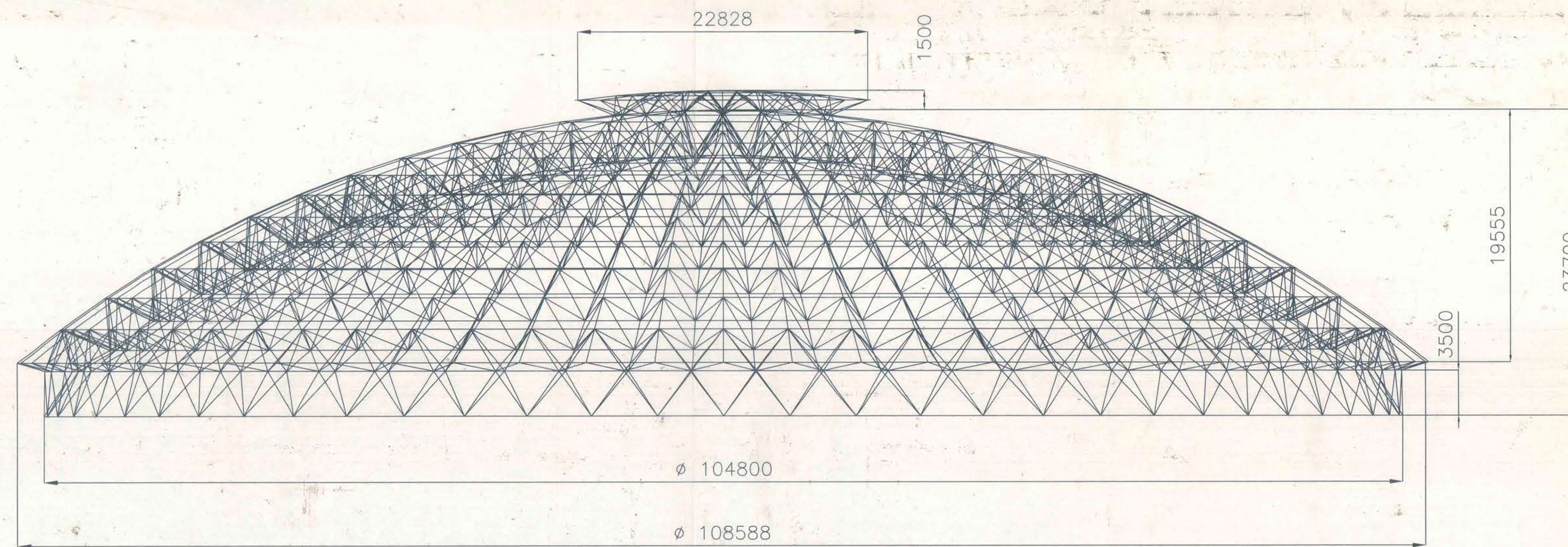
ELEVACION TIPO GEOMETRIA CUPULA ESCALA 1: 200
