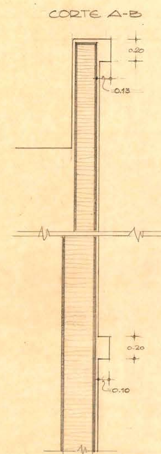
CORTE A-B
