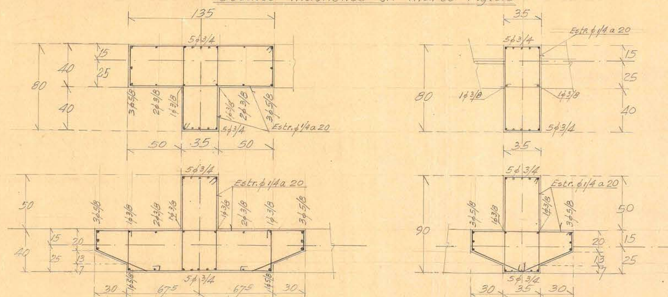
Detalle machones en marco rigido
