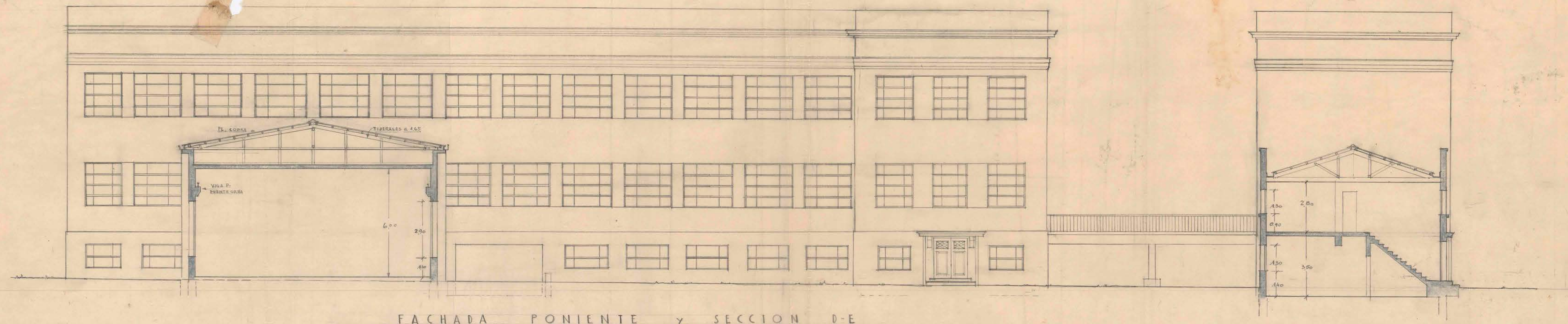
FACHADA PONIENTE y SECCION D-E
