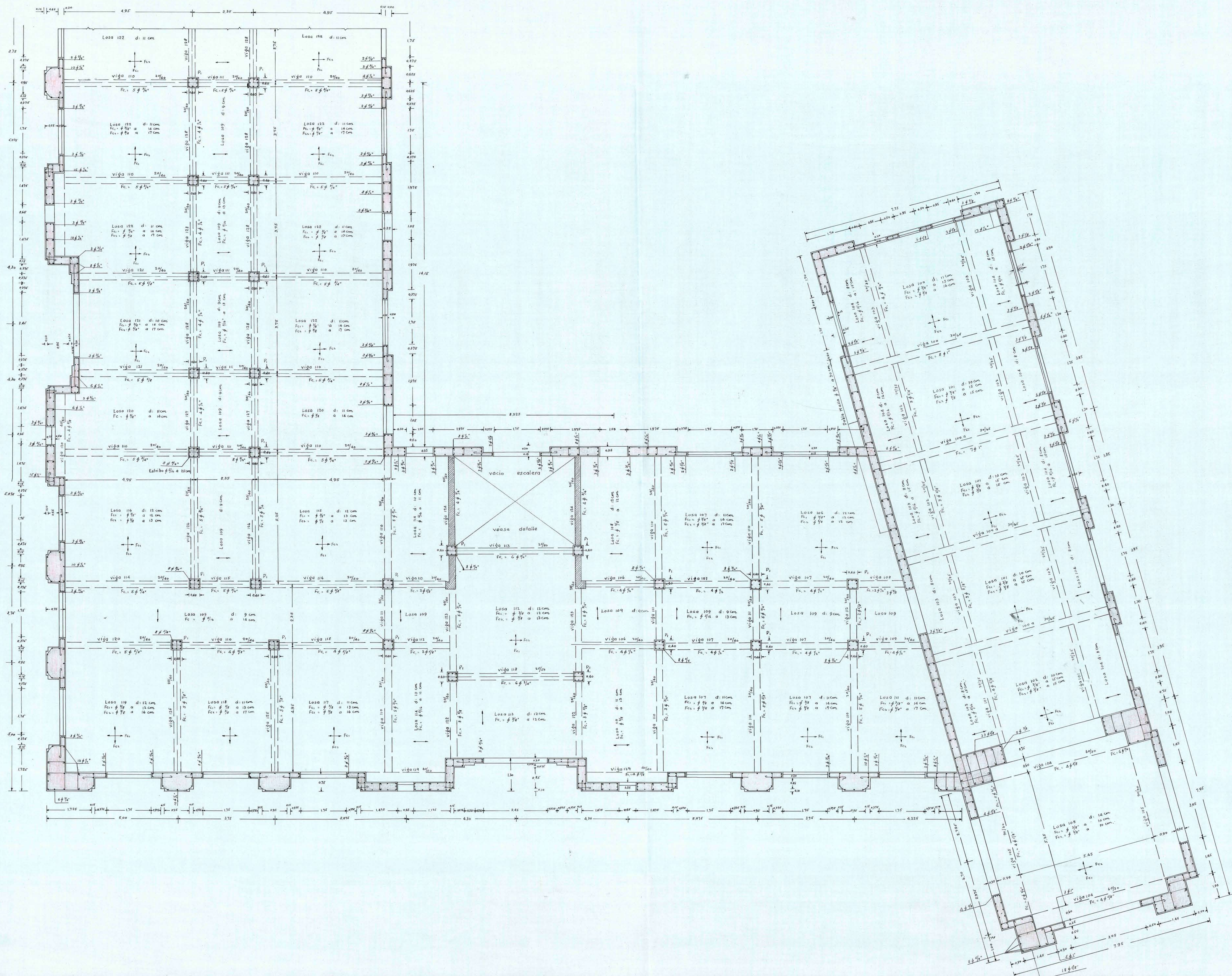
SUPERINTENDENCIA DE ADUANAS.- VALPARAISO.- CORTE HORIZONTAL POR EL 1º PISO VIGAS Y LOSAS EN EL SUELO 2º PISO.- ESCALA 1:50
