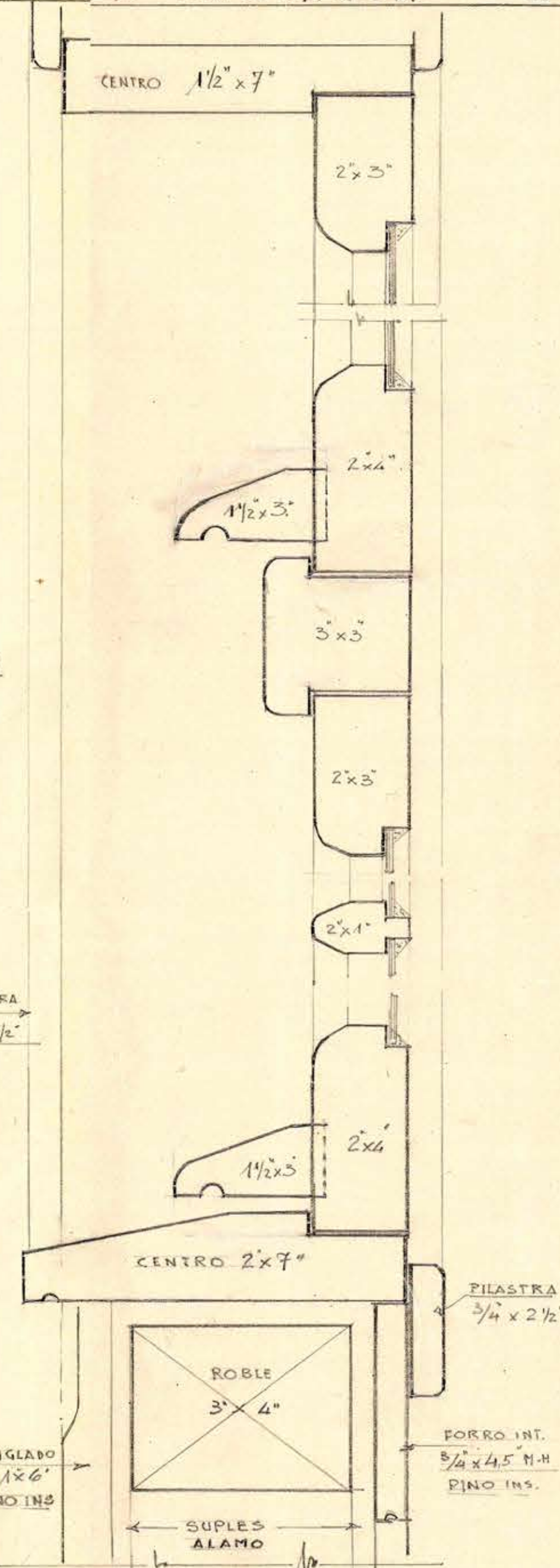
SECCION A-B TAMAÑO 1/2 NATURAL
