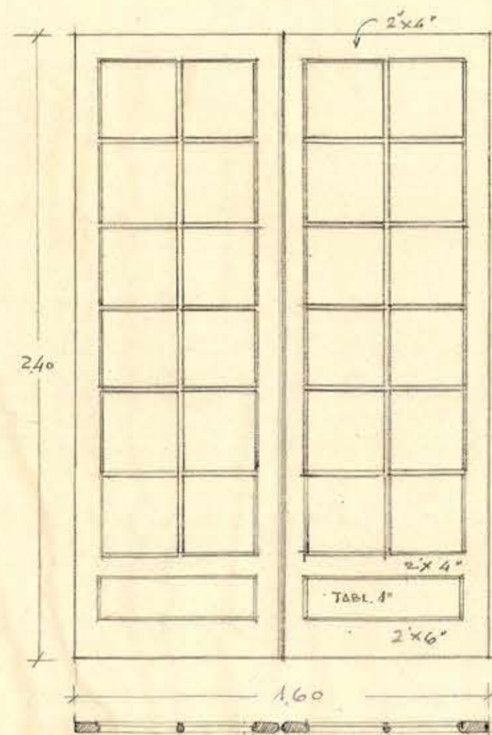
PUERTA DE VAIVEN (1)
