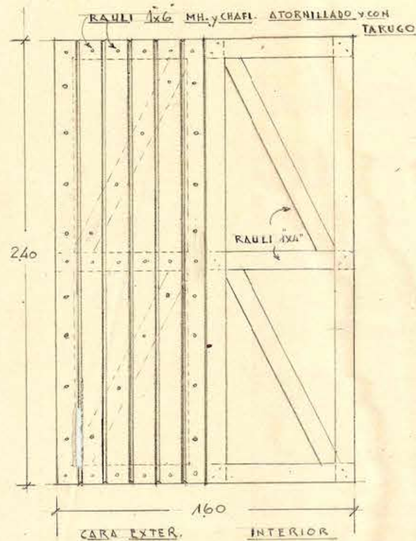
PUERTA DE FACHADA (2)
