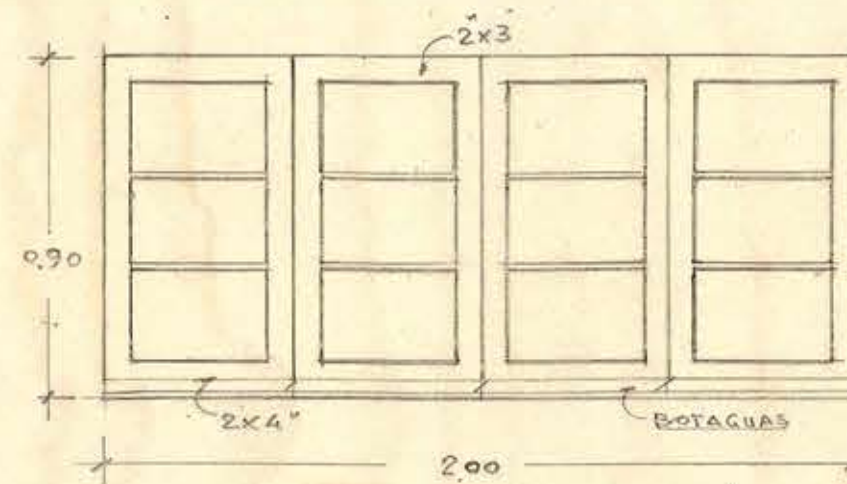
(2) VENTANAS DE LOS SERVICIOS HIGIEN. (2)
