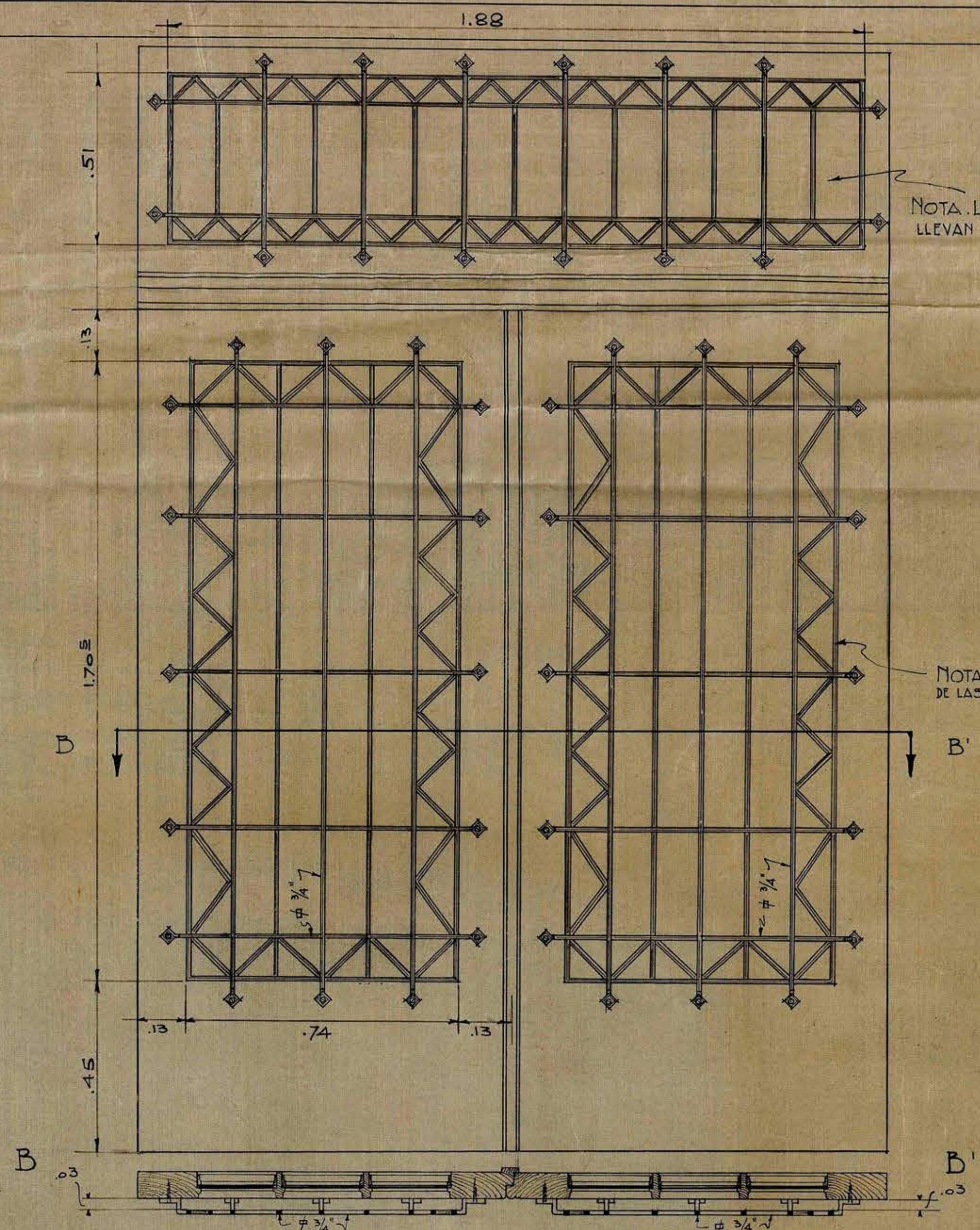
DETALLE DE LAS DEJAS DE FIERRO PARA LA PUERTA TIPO "A-A" DE LA ENTRADA PRINCIPAL Y DE LAS PUERTAS TIPO "A". ESCALA 1:10
