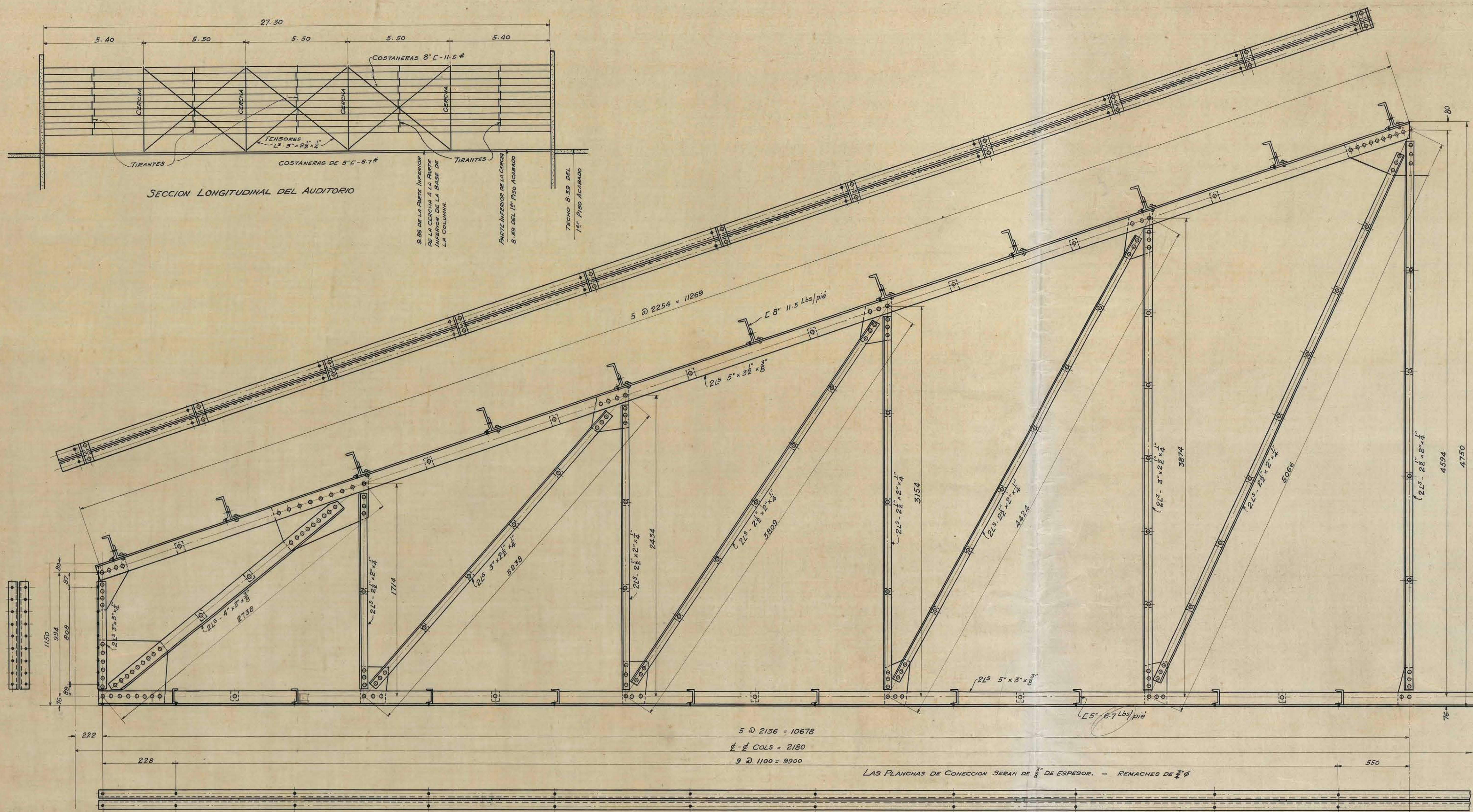
CERCHA - TRAMO 21.80 M. 4 POR AUDITORIO
