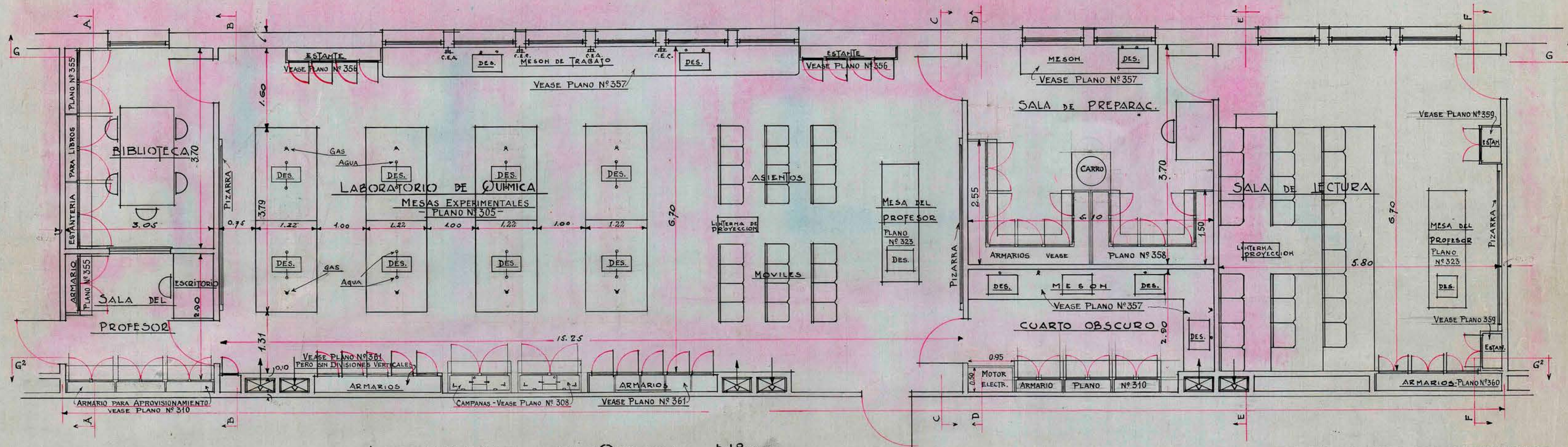
LABORATORIO DE QUIMICA N° 202 PARA 24 ALUMNOS ESCALA 0.02=1MTR.
