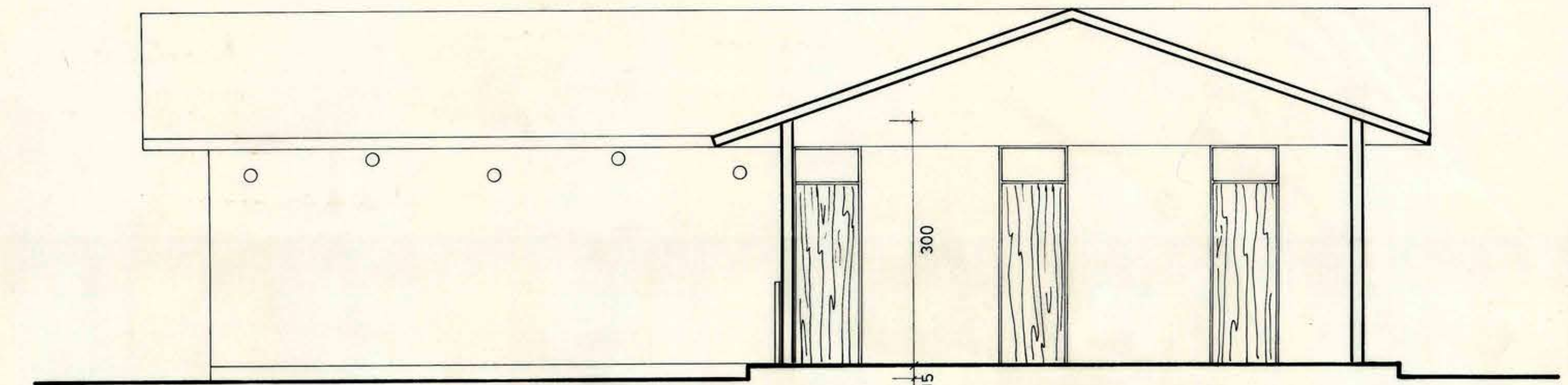
CORTE ELEVACION A-A
