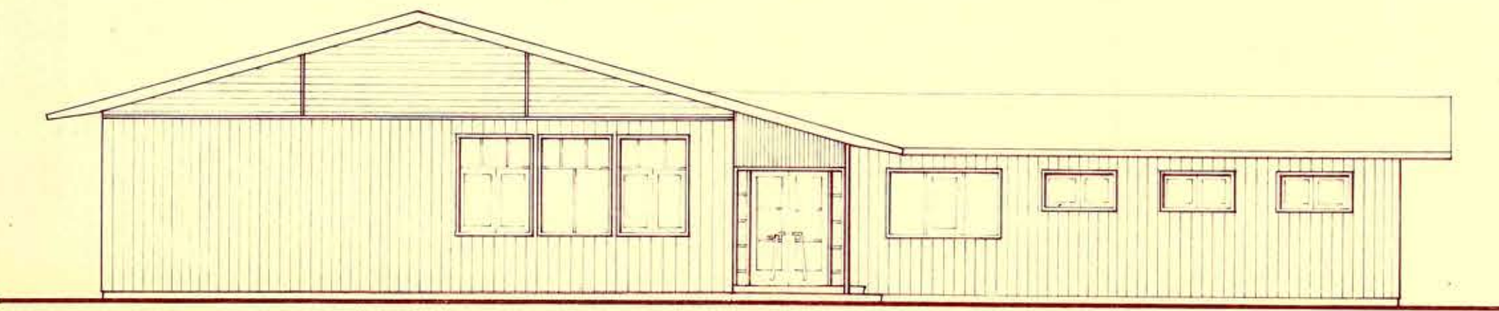
ELEVACION ORIENTE.
