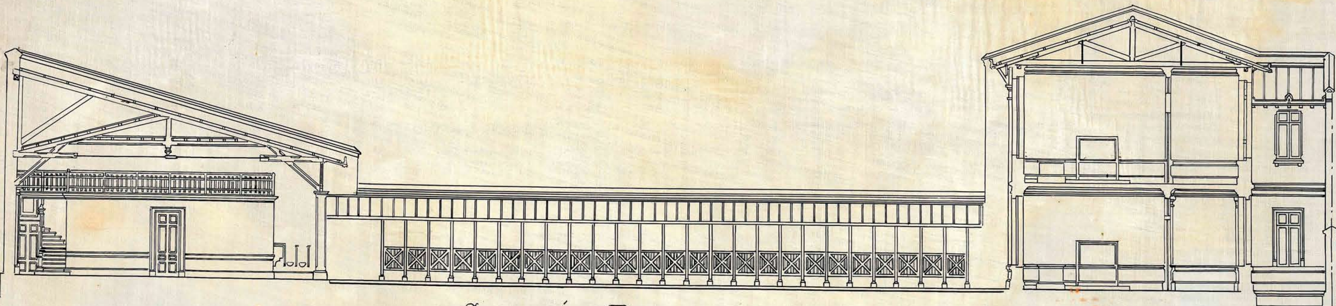
~ SECCION TRANSVERSAL ~
