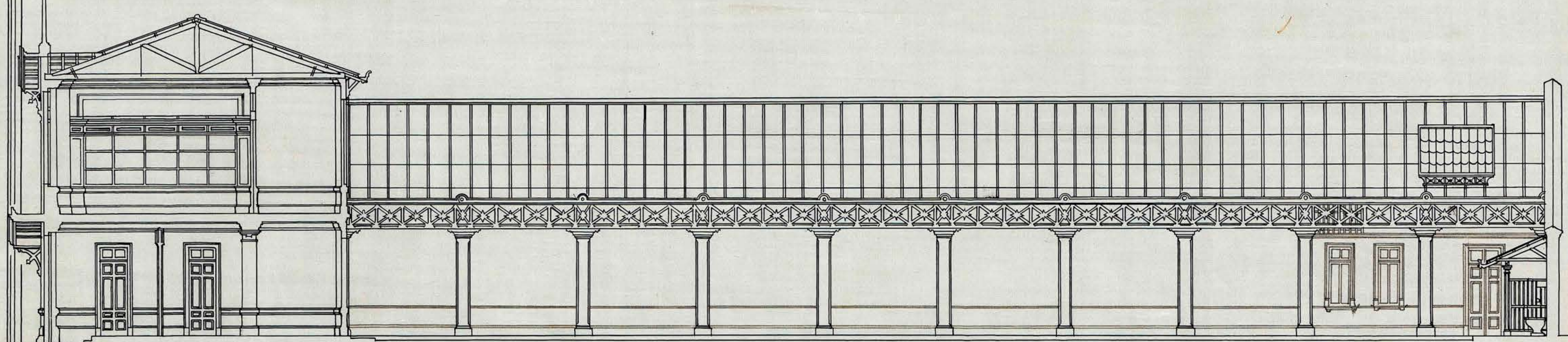
SECCION LONGITUDINAL.
