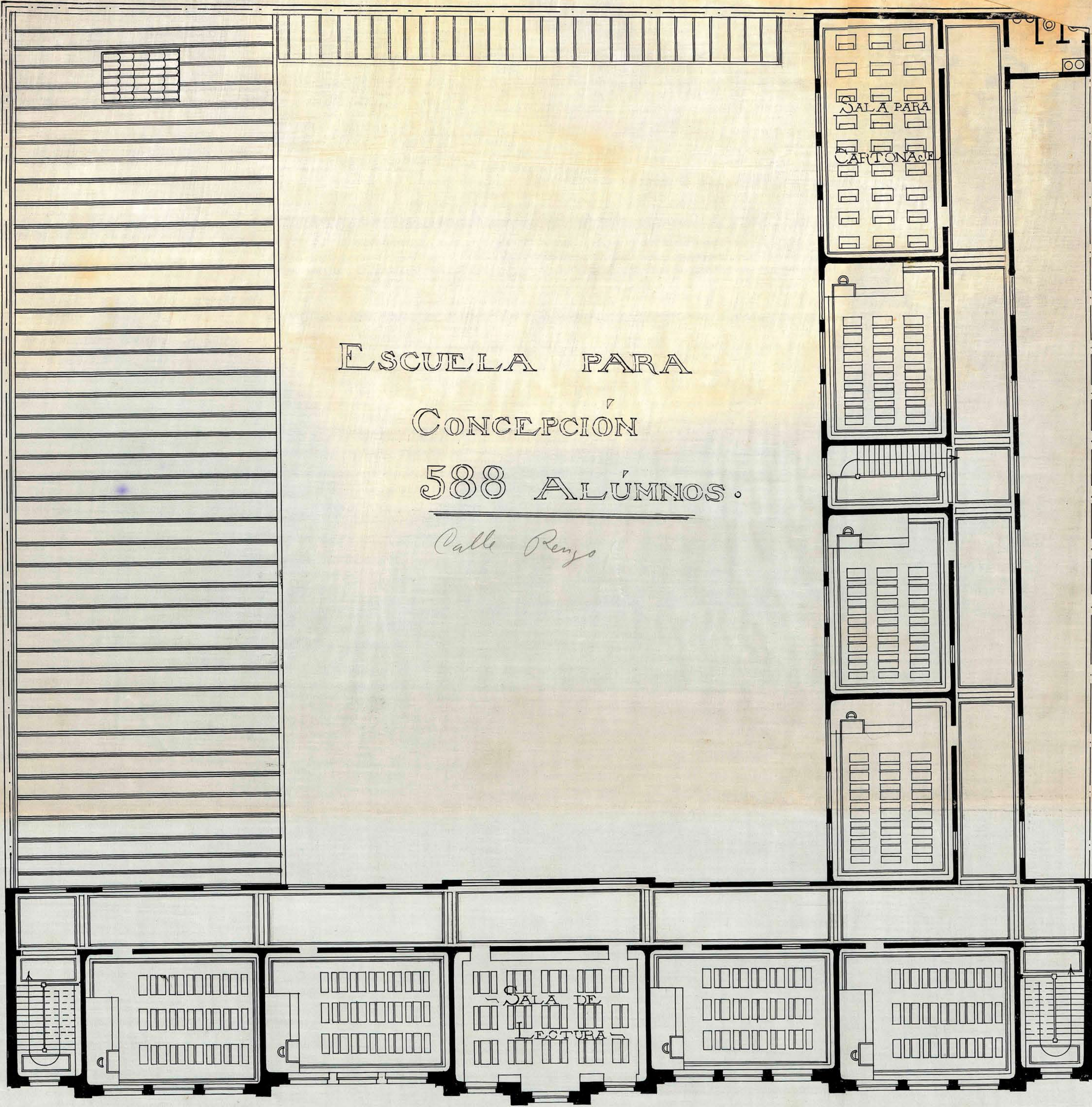
PLANO SEGUNDO PISO.
