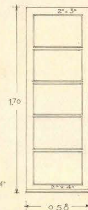
DETALLE DE LOS VENTANALES DE LA TECHUMBRE
