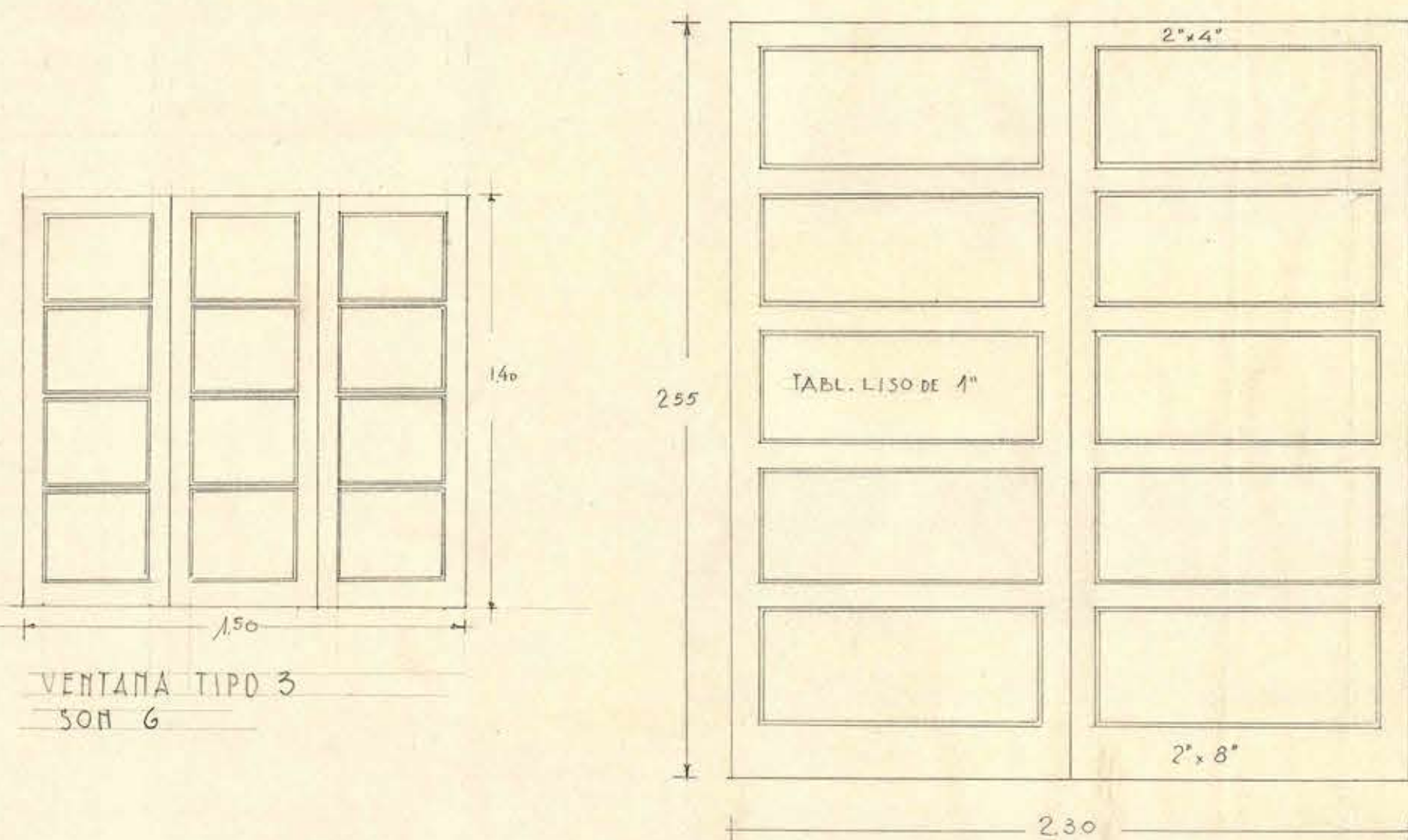
PUERTA TIPO A SON 6
