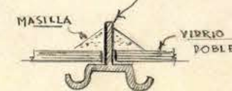
DETALLE DE LOS VENTANALES DE LA TECHUMBRE
