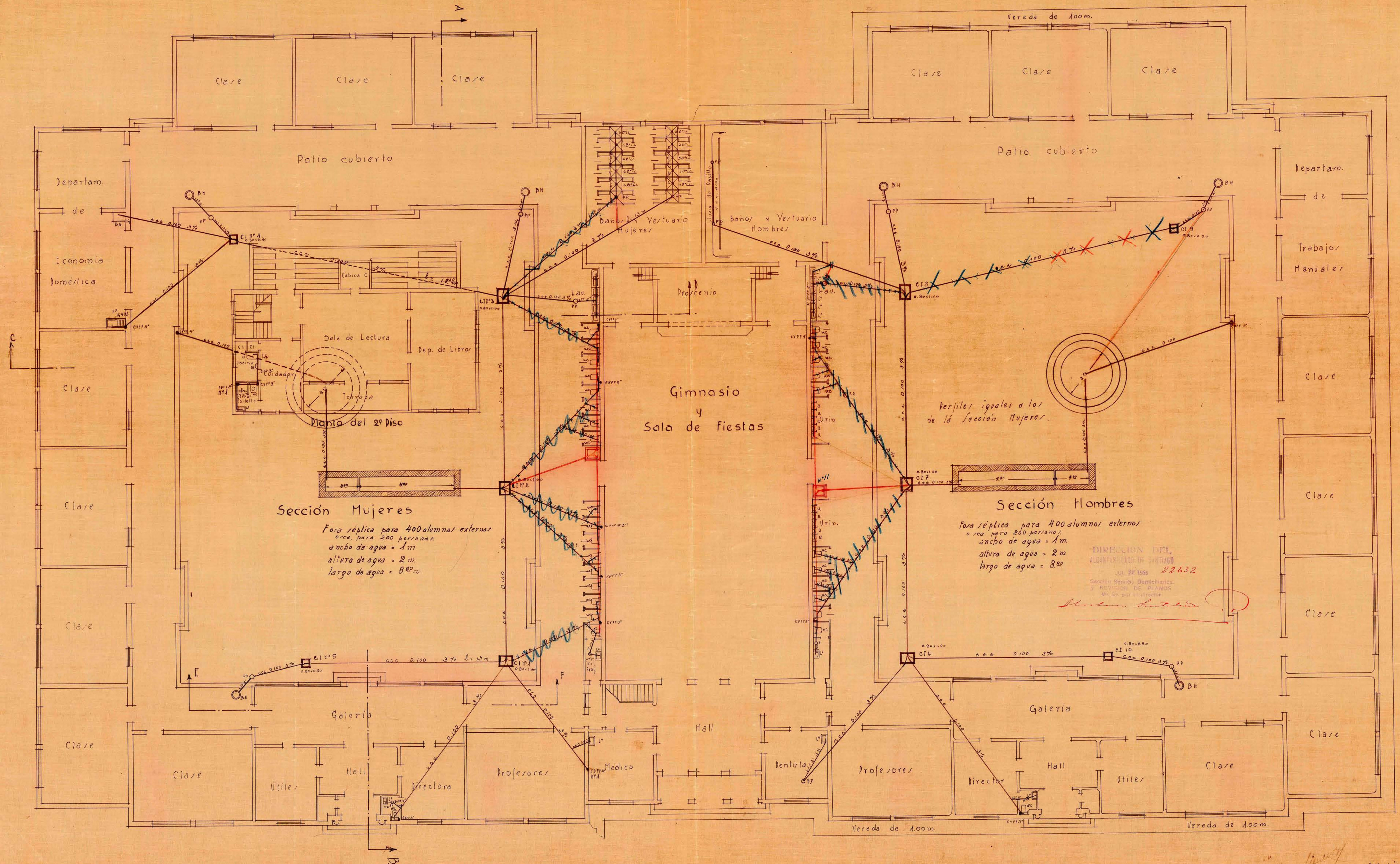
Planta del 1º Piso
