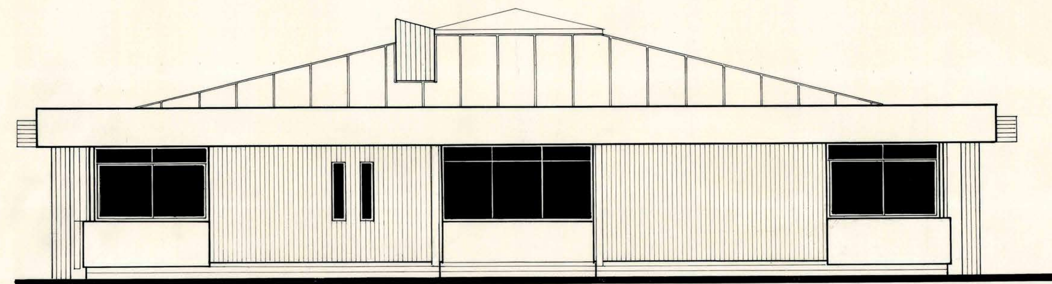
FACHADA NORTE
