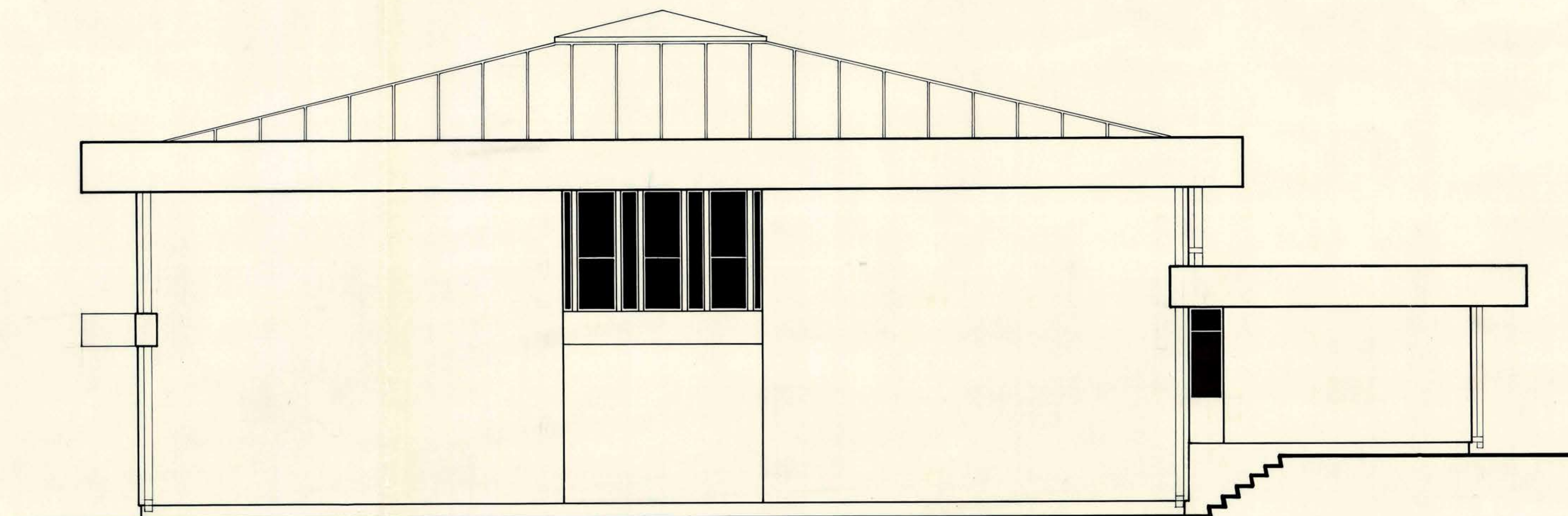
FACHADA NORTE (SUR)
