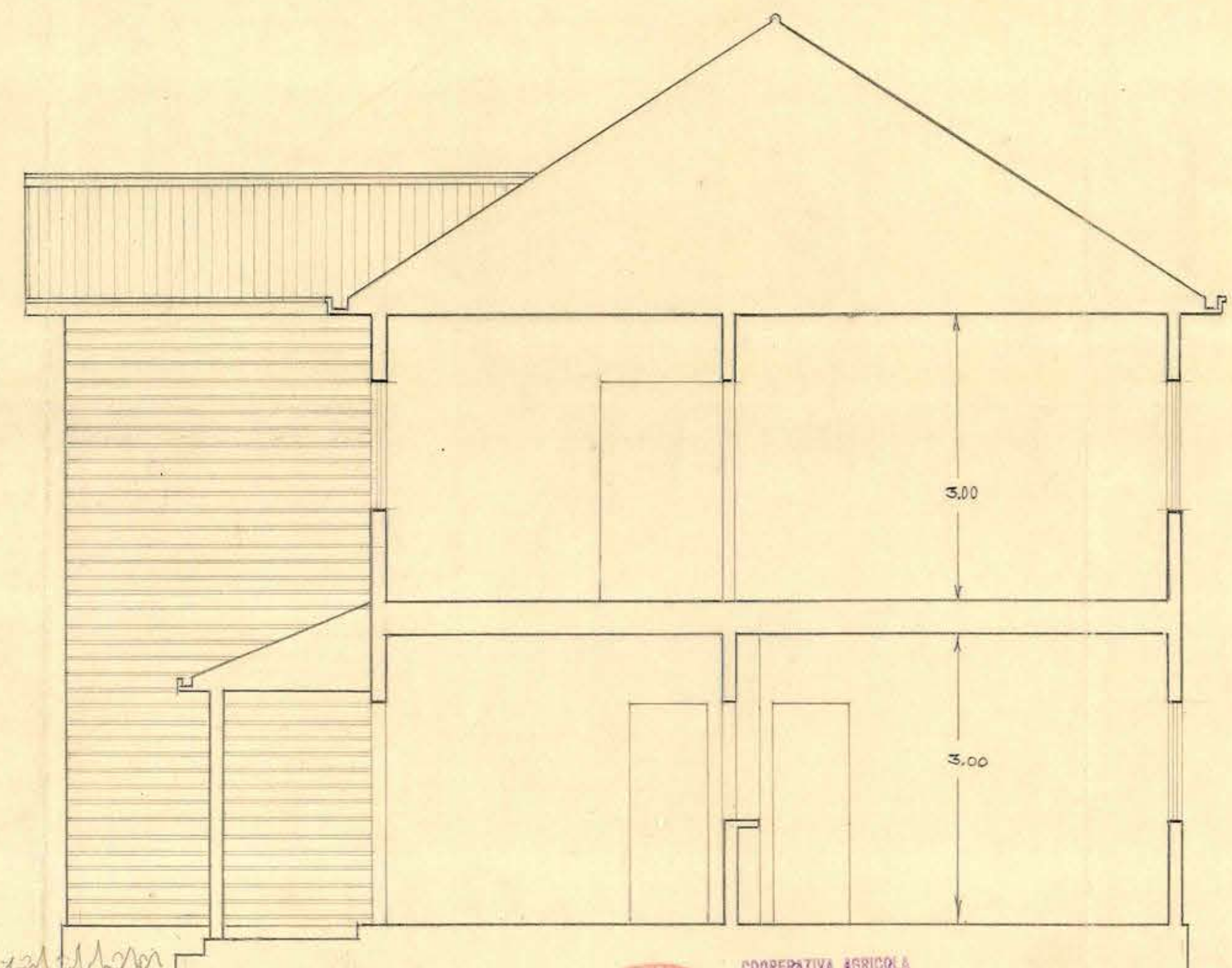
● CORTE AB
