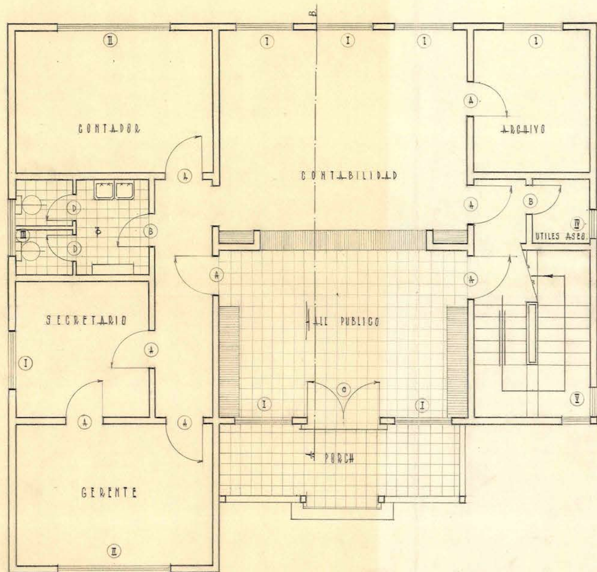
● PRIMER PISO
