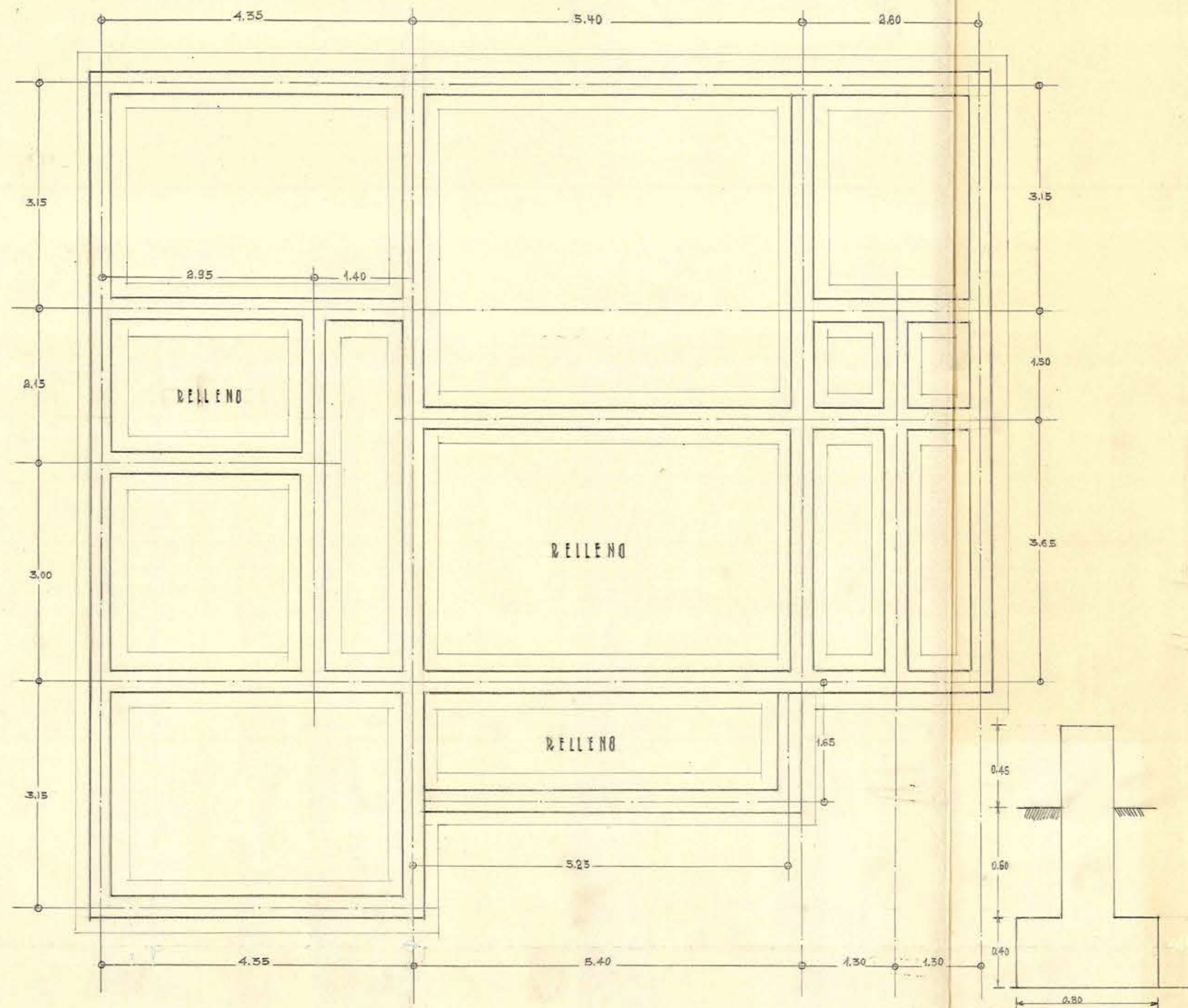
● PLANO CIMIENTOS
