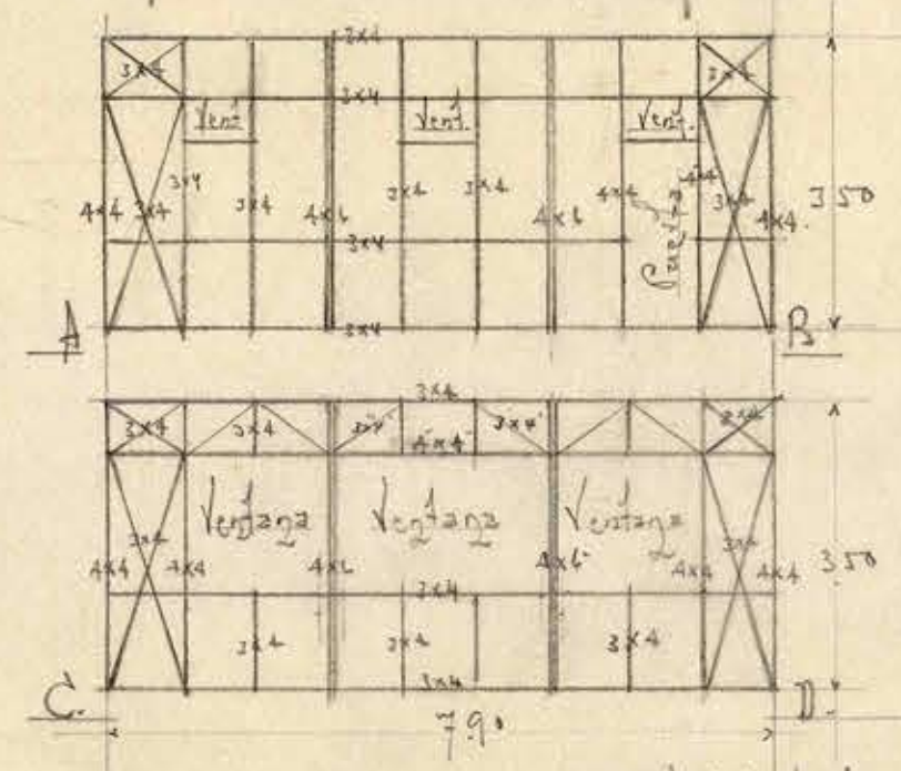
- Isograma entramado fabrique -
