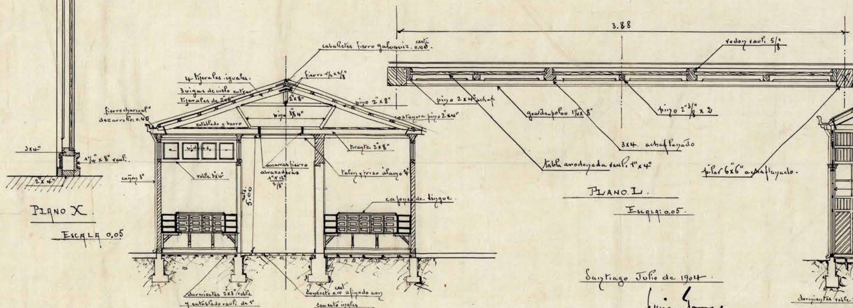
SECCION C.D.
