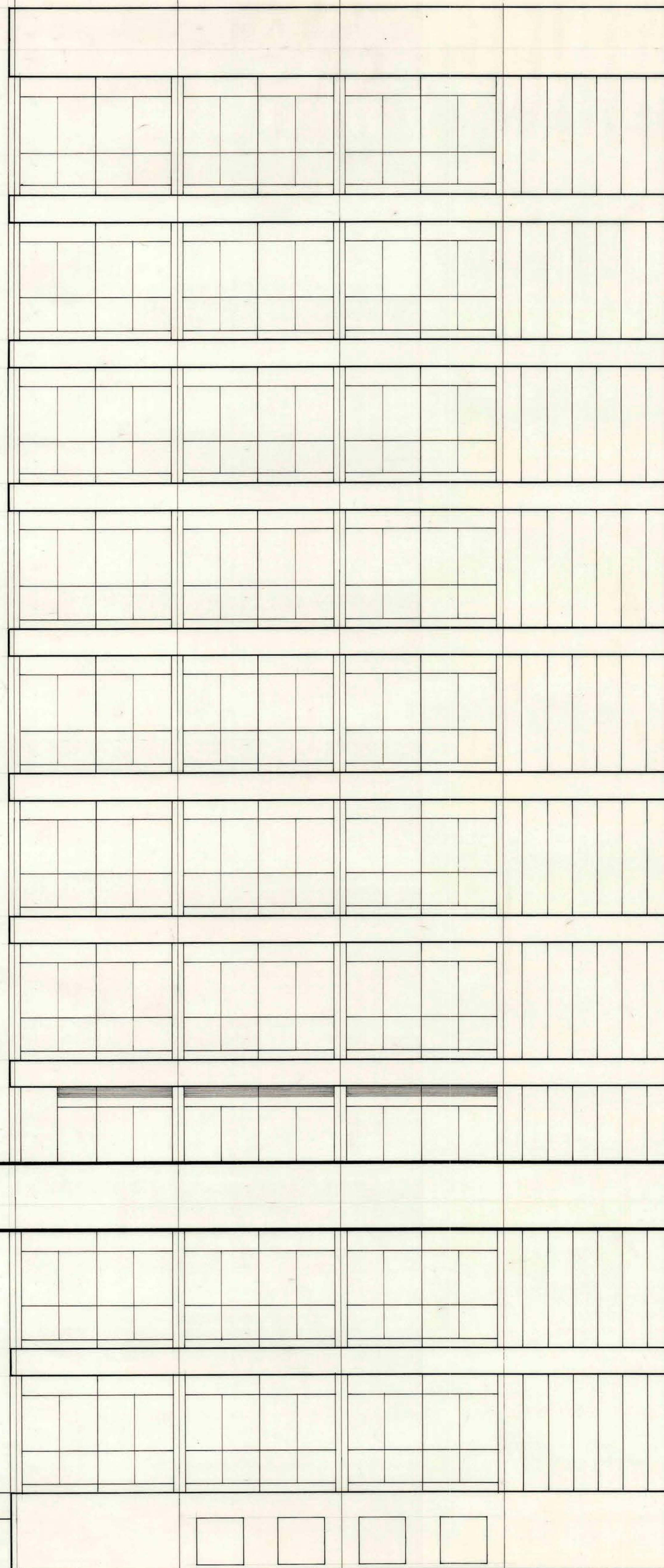
ELEVACION SUR
