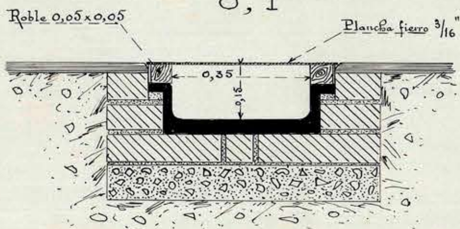
CORTE B. 0,1
